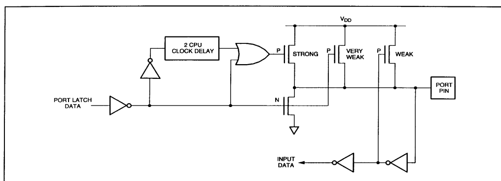
图 9 准双向口输出
