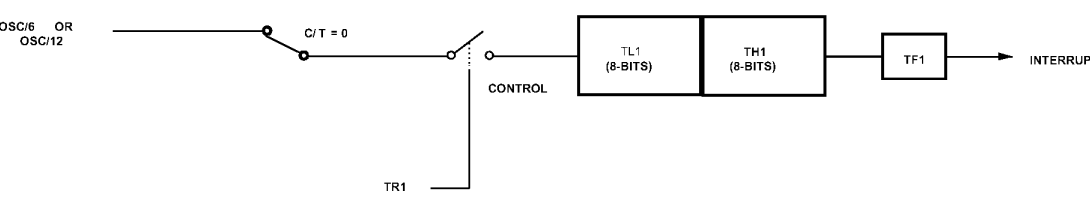
图 25 模式 1 时定时器 1 (16 位定时器)
