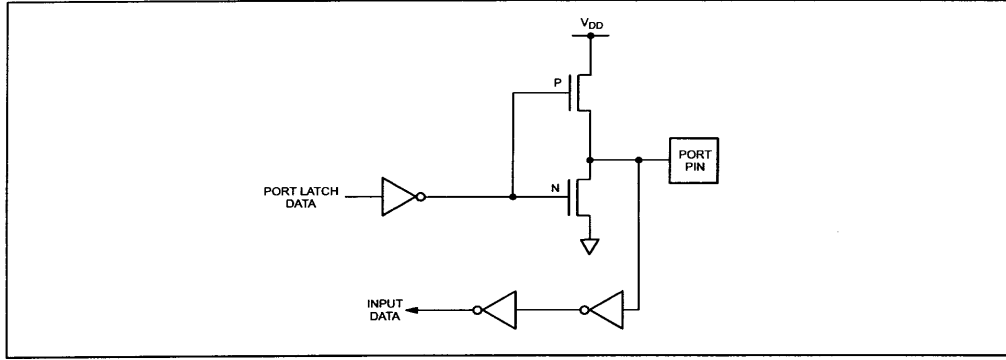
图 11 推挽输出
