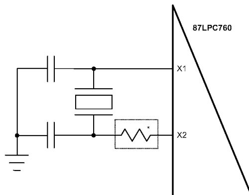
图 15 晶振的使用
