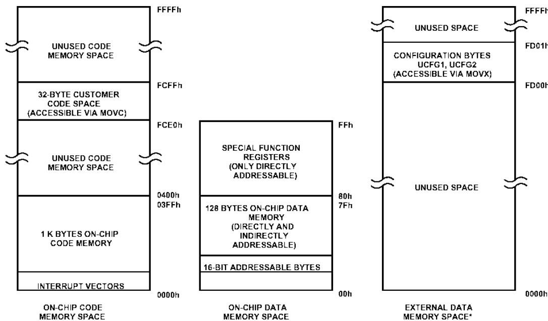
图 1 P87LPC760 程序和数据存储器分布图
