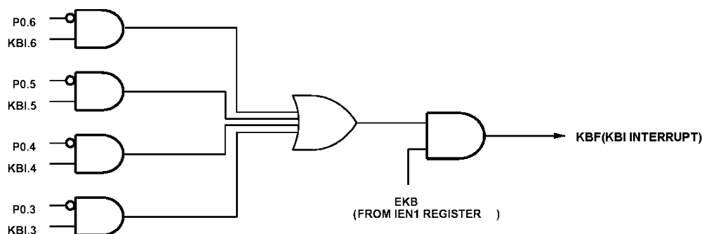
图 13 键盘中断
