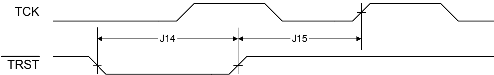
图 21-10. JTAG TRST时序
