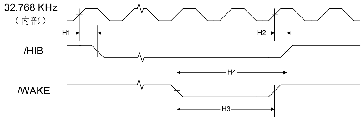
图 21-4. 休眠模块时序
