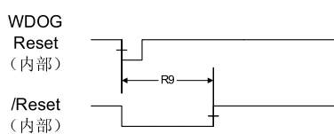
图 21-15. 看门狗复位时序
