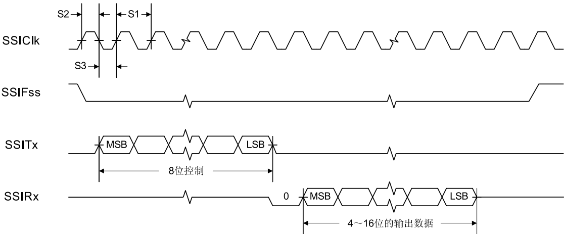
图 21-6. MICROWIRE 帧格式 (FRF=10) 的 SSI 时序, 单次传输
