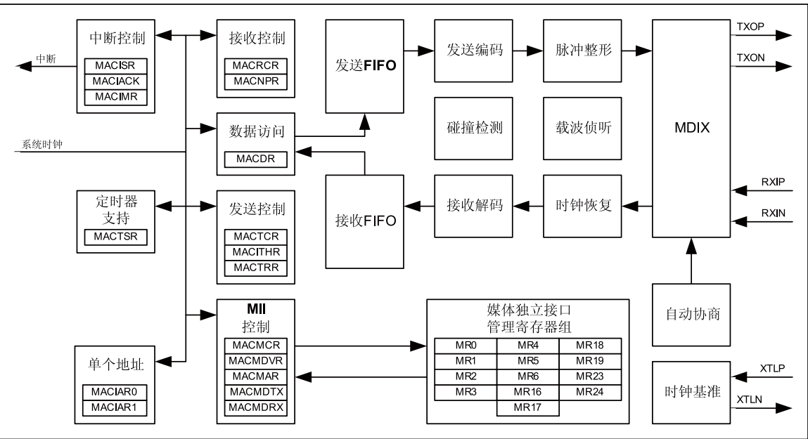
图 16-1. 以太网控制器方框图
