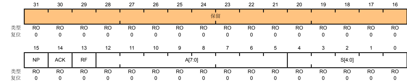
以太网PHY管理寄存器5 – 自协商连接方基页能力 (MR5) 类型 RO, 复位 0x0000
