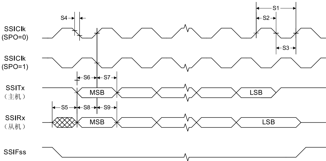
图 21-7. SPI 帧格式 (FRF=00), SPH=1
