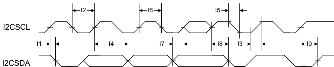
图 21-2. I 2 C时序
