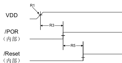
图 21-13. 掉电复位时序
