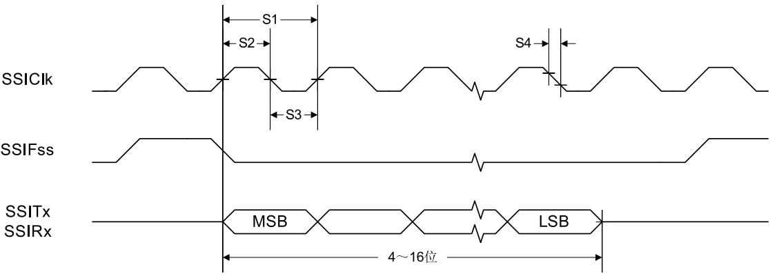
图 21-5. TI帧格式 (FRF=01) 的SSI时序，单次传输的时序测量
