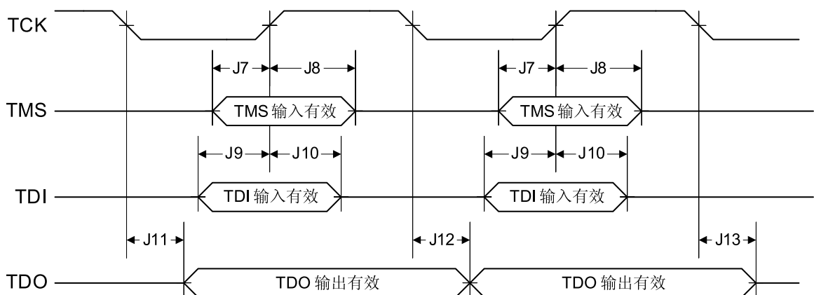
图 21-9. JTAG测试访问端口 (TAP) 时序
