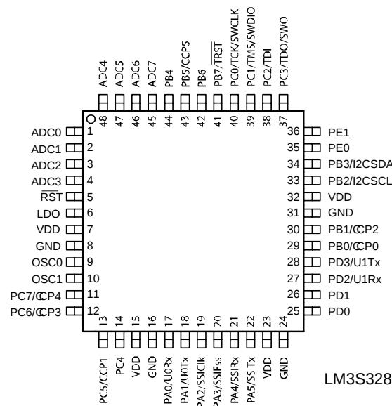
图 2.1 管脚连接图
