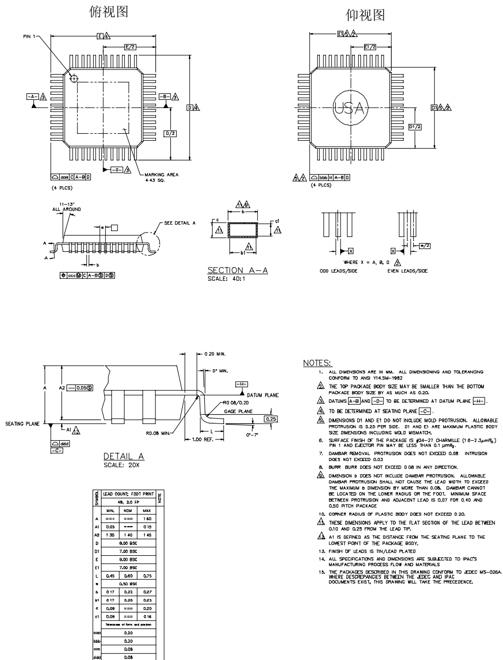
图 4.1 48 脚 LQFP 封装
