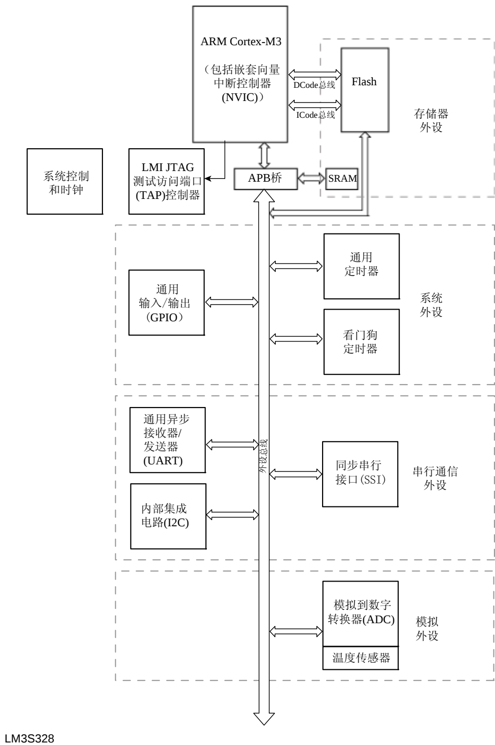
图 1.1 Stellaris 高级方框图
