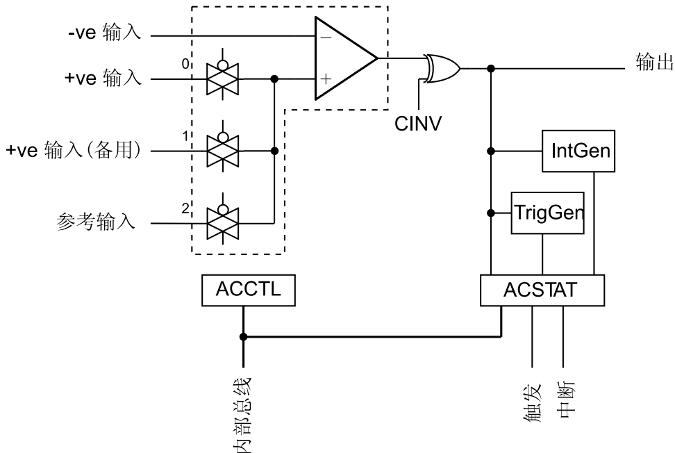
图 17-2. 比较单元的结构
