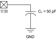
图 21-1. 负载条件
