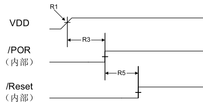
图 21-12. 掉电复位时序
