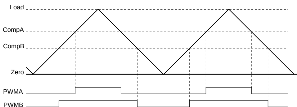
图 16-4. 在先递增后递减计数模式中产生PWM信号
