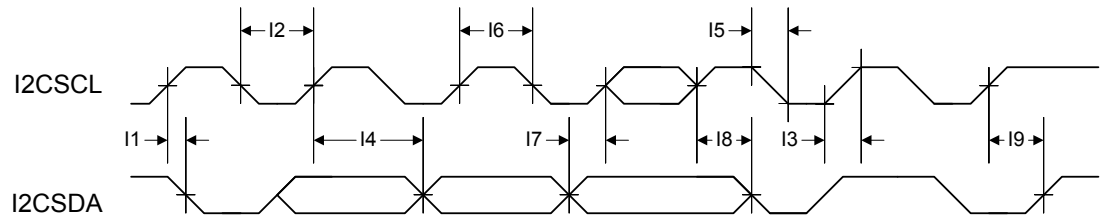
图 21-2. I 2 C时序
