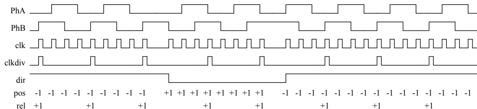
图 17-2. 正交编码器和速度预分频器的操作
