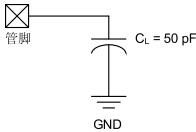
图 21-1. 负载条件
