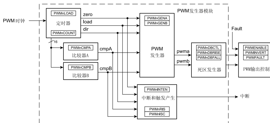
图 16-1. PWM 模块的结构图
