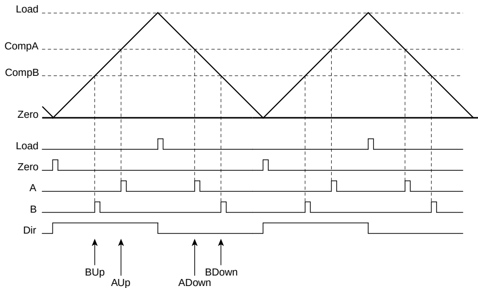
图 16-3. PWM先递增后递减计数模式
