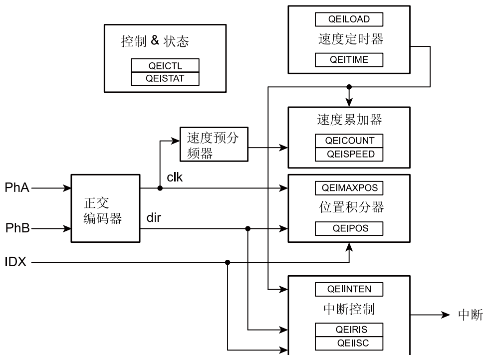
图 17-1. QEI结构图
