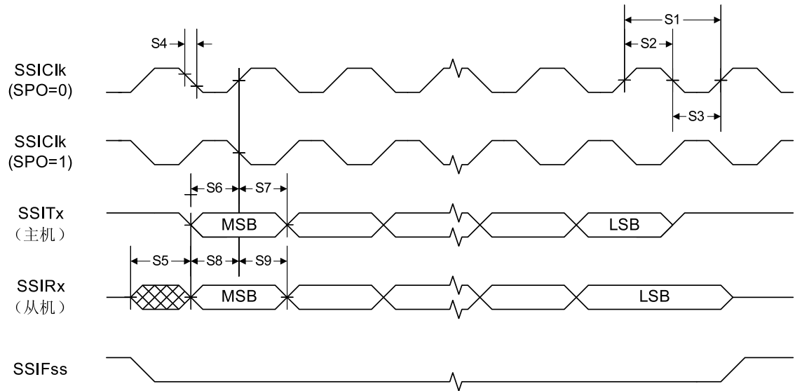
图 21-6. SPI 帧格式 (FRF=00), SPH=1
