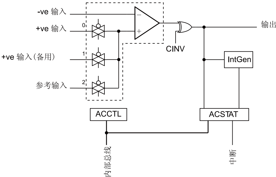
图 15-2. 比较单元的结构
