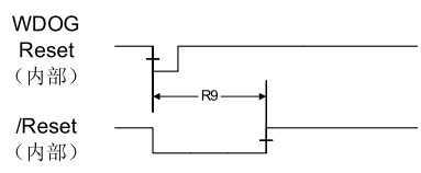
图 21-14. 看门狗复位时序
