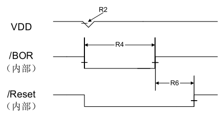
图 21-12. 掉电复位时序
