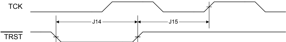
图 21-9. JTAG TRST时序
