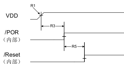
图 21-11. 上电复位时序
