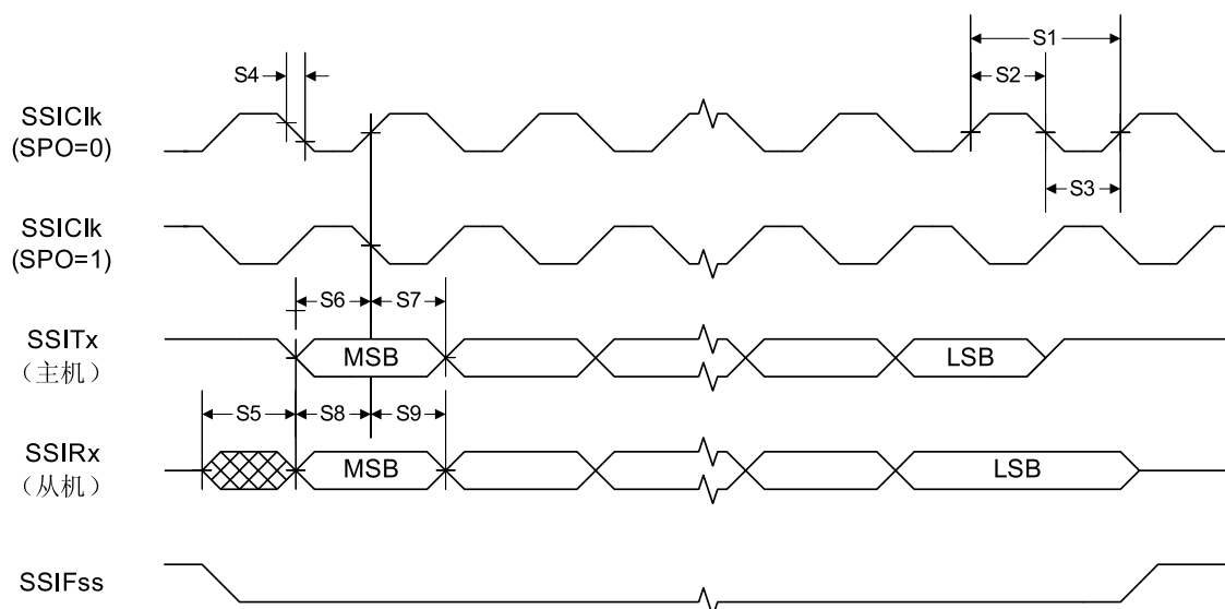
图 21-6. SPI 帧格式 (FRF=00), SPH=1
