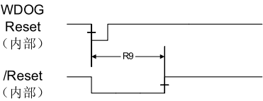
图 21-14. 看门狗复位时序
