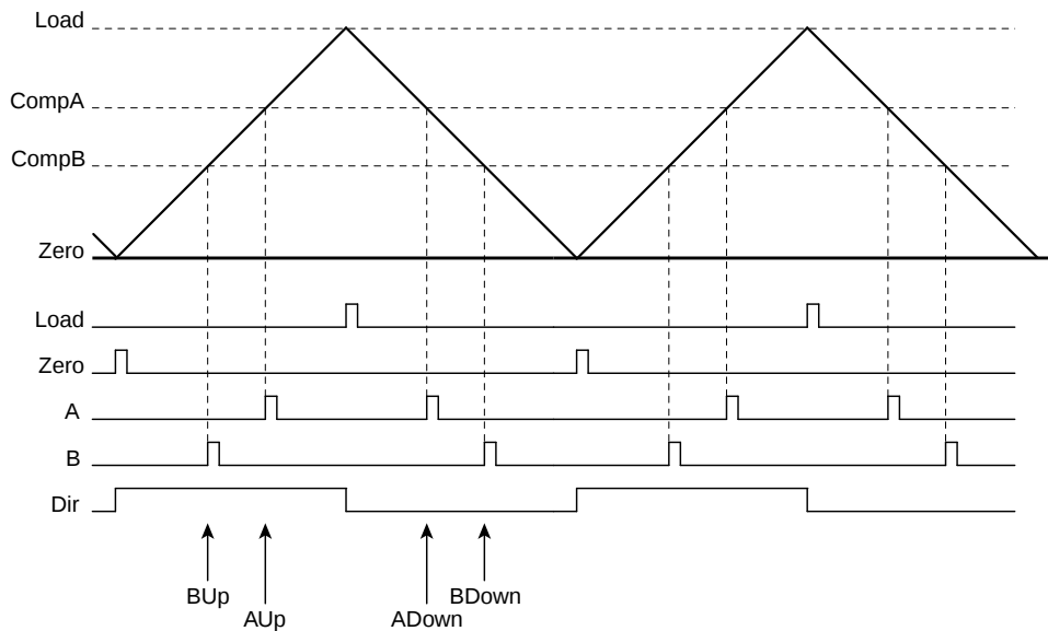
图 17-3. PWM先递增后递减计数模式
