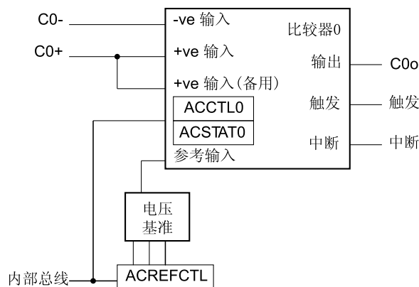
图 16-1. 模拟比较器模块的结构图
