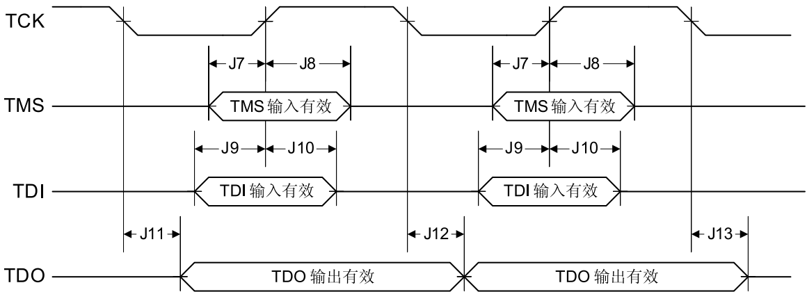
图 21-8. JTAG测试访问端口（TAP）时序
