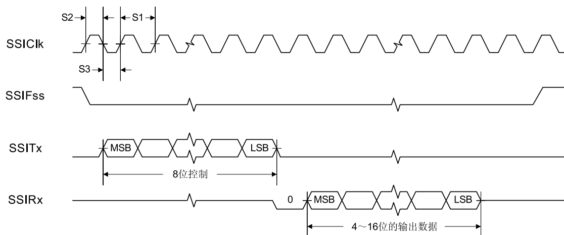
图 21-5. MICROWIRE 帧格式 (FRF=10) 的 SSI 时序, 单次传输
