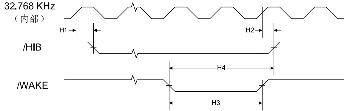
图 21-3. 休眠模块时序
