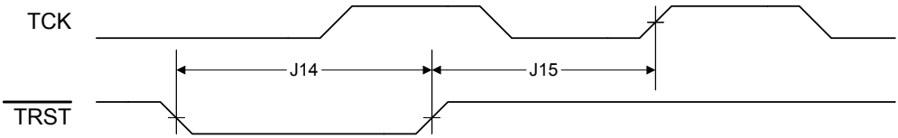
图 21-9. JTAG TRST时序
