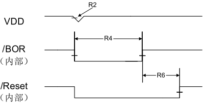
图 21-13. 软件复位时序
