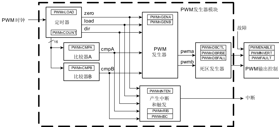
图 17-1. PWM模块的结构图
