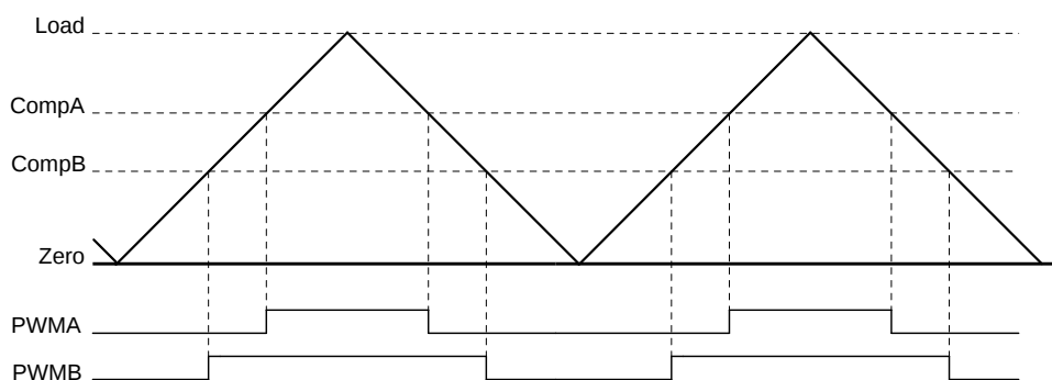
图 17-4. 在先递增后递减计数模式中产生PWM信号
