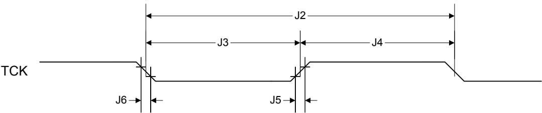
图 21-7. JTAG测试时钟输入时序
