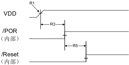
图 21-12. 掉电复位时序
