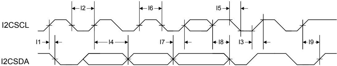
图 21-2. I 2 C时序
