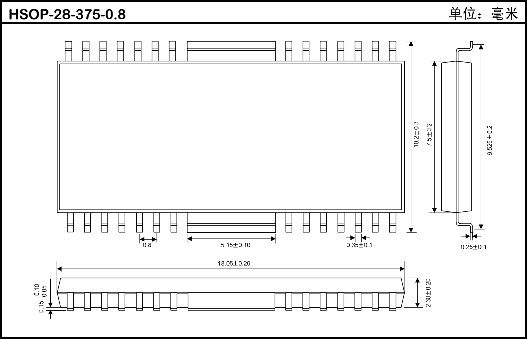
封装外形图
