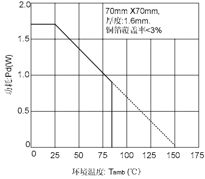
图1. 热功耗曲线
