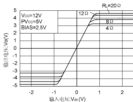
图3. 驱动器输入/输出特性 (sled)
