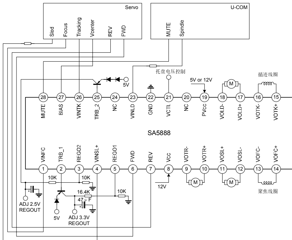
典型应用电路图
