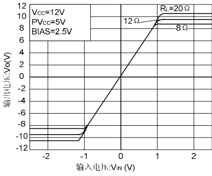
图2. 驱动器输入/输出特性 (Spindle)
