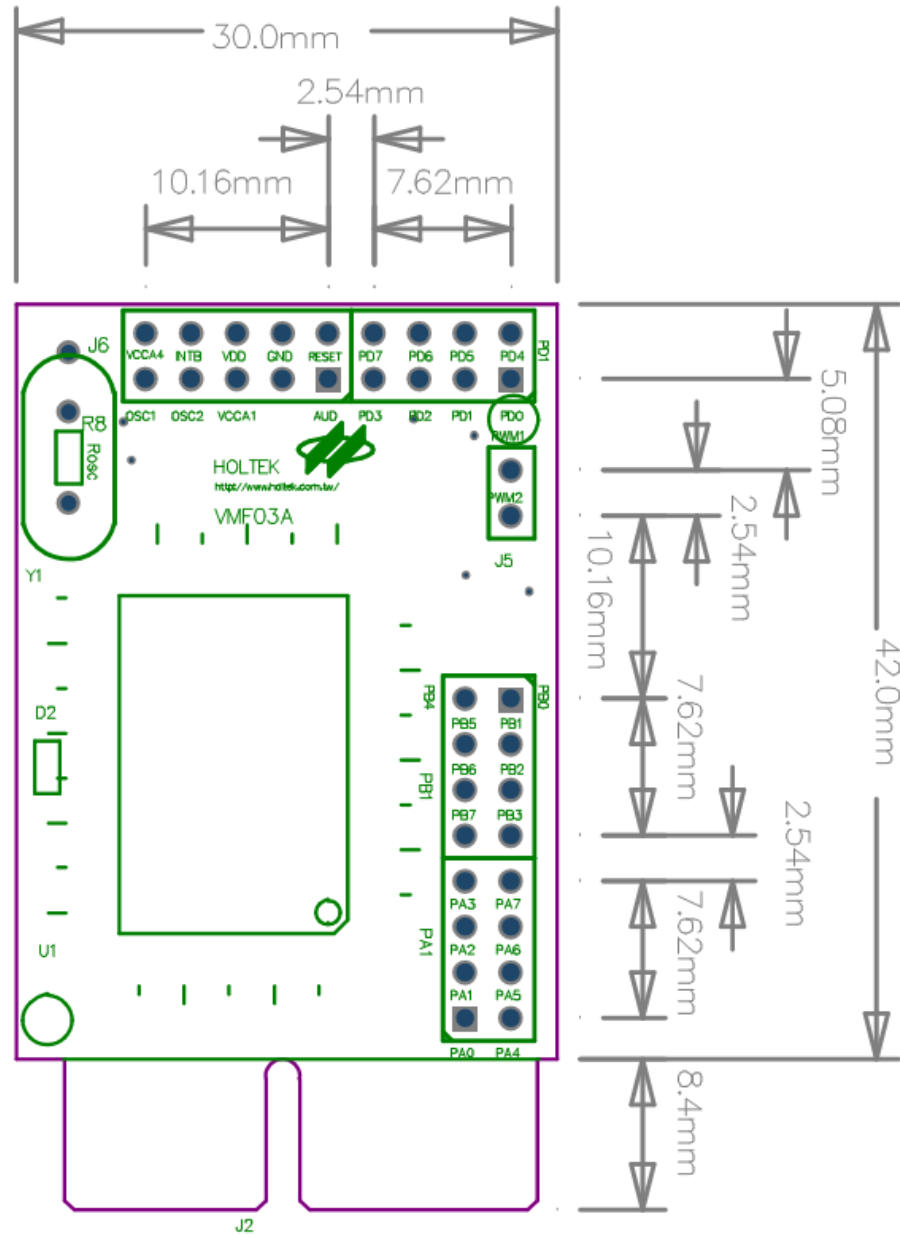
VMF03A 尺寸圖
