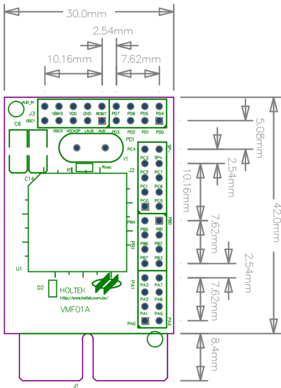
VMF01A 尺寸圖
