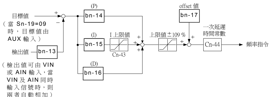
圖 12 PID 控制方塊圖
