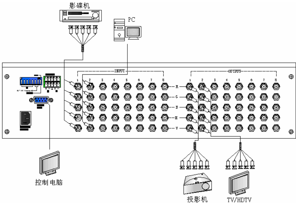
图 5-1 BX 矩阵系统接线图
