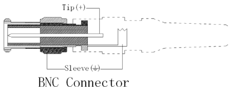
图 5-2 BNC 接线示意图
