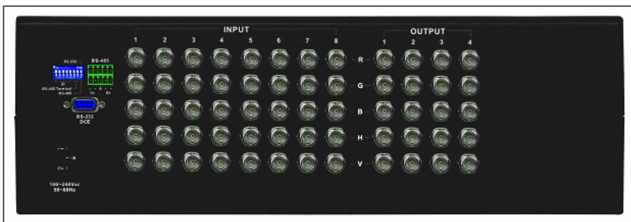
图 4-4 BX-3084 后面板示意图
