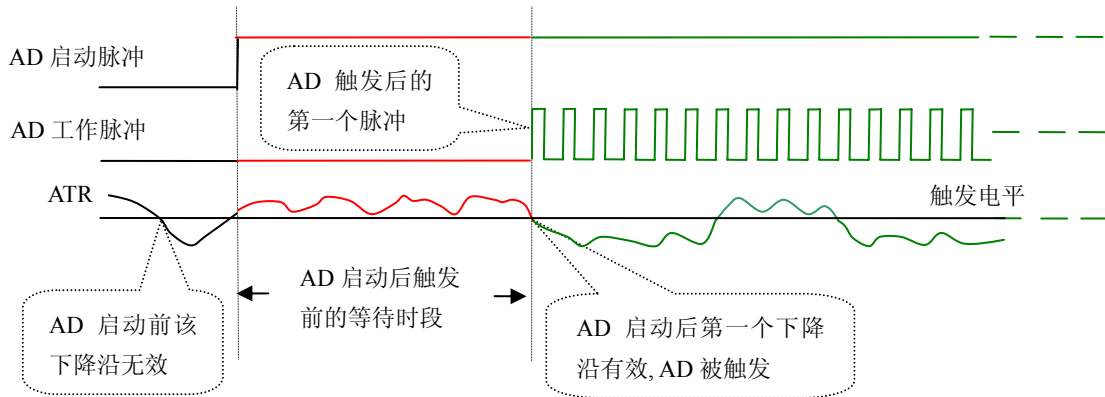
图 7.3 下降沿触发图例，上升沿同理
