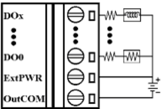
集电极输出接线图
