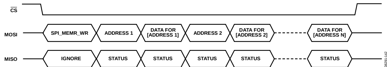
图94. 存储器（MCR、BBRAM或包RAM）随机地址写入
