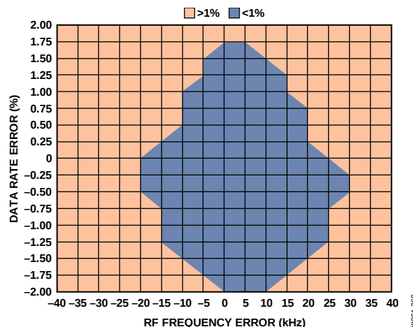
图64. AFC关闭：误包率与RF频率误差和数据速率误差的关系， AFC关闭, 数据速率=300 kbps, 频率偏差 = 75 kHz, GFSK, AGC_LOCK_MODE = 前同步码后锁定
