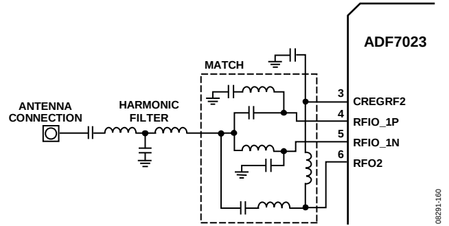
图112. 合并单端PA和LNA匹配
