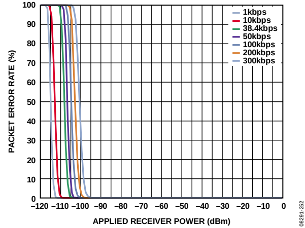
图 56. 误包率与RF输入功率和数据速率的关系：FSK/GFSK、928 MHz、 前同步码长度 = 64位、 V_{DD} = 3.0 V、温度 = 25°C
