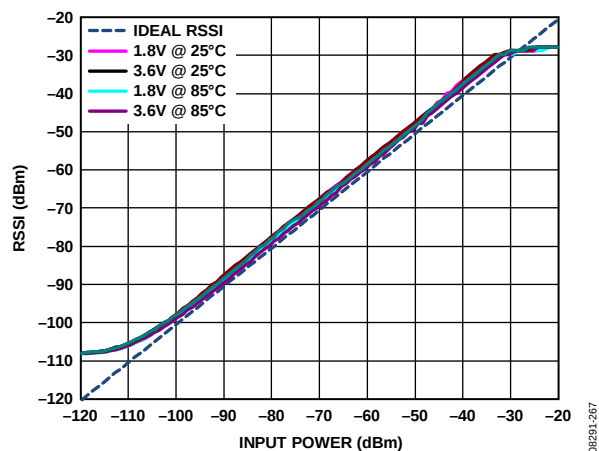
图71. OOK RSSI与RF输入功率、 V_{DD} 和温度的关系： RF频率 = 915 MHz， 数据速率 = 19.2 kbps (38.4 kbps曼彻斯特编码)
