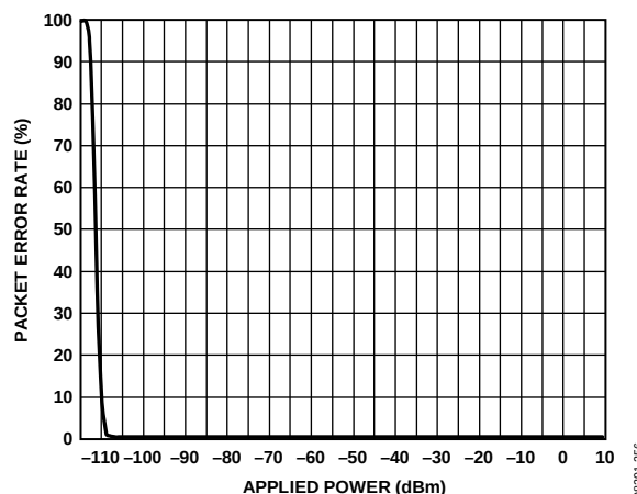
图59. OOK误包率与RF输入功率的关系：数据速率 = 19.2 kbps (芯片速率 = 38.4 kcps, 曼彻斯特编码), IF带宽 = 100 kHz, V_{DD} = 3.6 V, 温度 = 25°C, RF频率 = 902 MHz, 前同步码长度 = 100位
