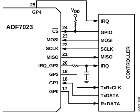
图111. Sport模式下的处理器接口
