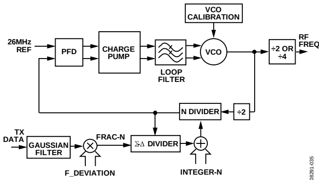
图106. RF频率合成器架构
