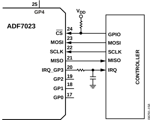
图110. 包模式下的处理器接口
