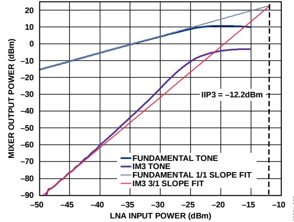
图32. LNA/混频器IIP3: V_{DD} = 3.0\text{ V} , 温度 = 25^{\circ}\text{C} , RF频率 = 915 MHz, LNA增益 = 高, 混频器增益 = 高, 信号源1频率 = (915 + 0.4)\text{ MHz} , 信号源2频率 = (915 + 0.7)\text{ MHz}
