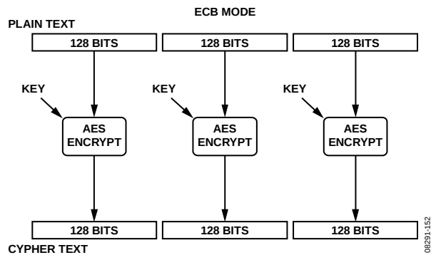
图104. ECB模式
