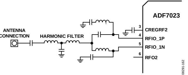
图114. 合并差分PA和LNA匹配
