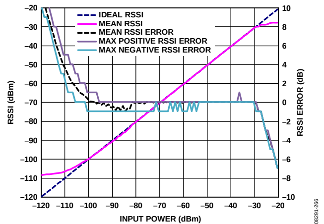
图70. OOK RSSI和OOK RSSI误差与RF输入功率的关系： 915 MHz，数据速率 = 19.2 kbps (38.4 kcps)， 每个输入功率电平进行200次RSSI测量
