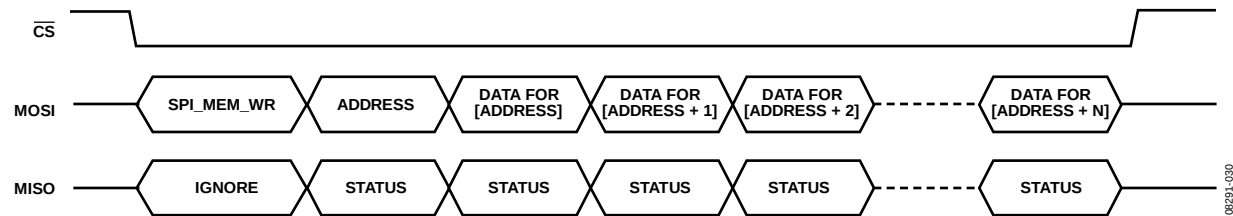
图93. 存储器（MCR、BBRAM或包RAM）块写入
