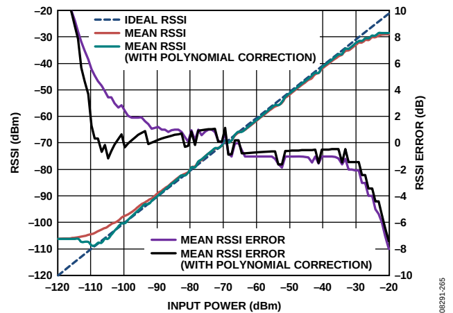
图69. 采用和不采用余弦多项式校正的RSSI （通过“自动包结束RSSI测量”）， 每个输入功率电平进行100次RSSI测量
