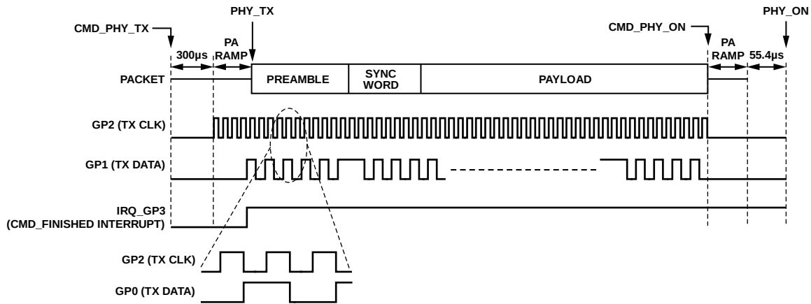
图81. Sport模式发送
