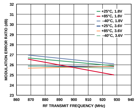
图28. 调制误差比(MER)与RF频率、温度和 V_{DD} 的关系, 调制指数 = 0.5, 数据速率 = 10 kbps
