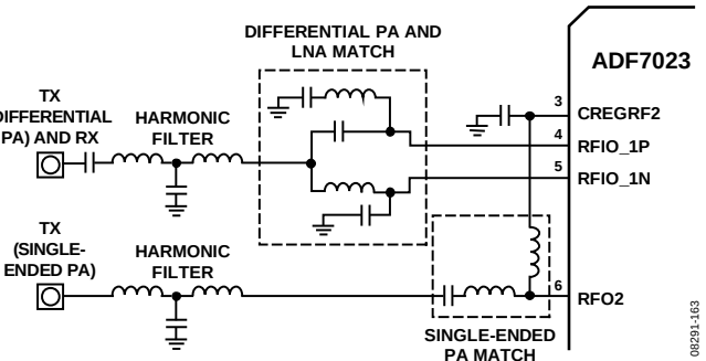
图115. 发射天线分集的匹配拓扑
