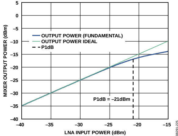
图29. LNA/混频器1 dB压缩点: V_{DD} = 3.0\text{ V} , 温度 = 25^{\circ}\text{C} , RF频率 = 915 MHz, LNA增益 = 低, 混频器增益 = 低
