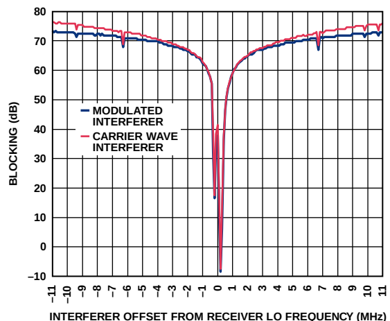
图41. 接收机宽带阻塞: 915 MHz、 数据速率 = 38.4 kbps
