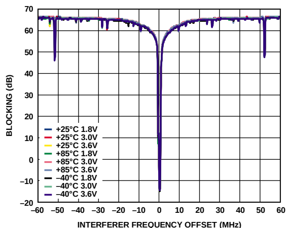
图44. 接收机宽带阻塞与 V_{DD} 和温度的关系: 915 MHz、 数据速率 = 300 kbps
