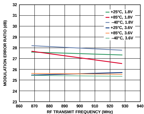
图26. 调制误差比(MER)与RF频率、温度和 V_{DD} 的关系, 调制指数 = 1, 数据速率 = 10 kbps
