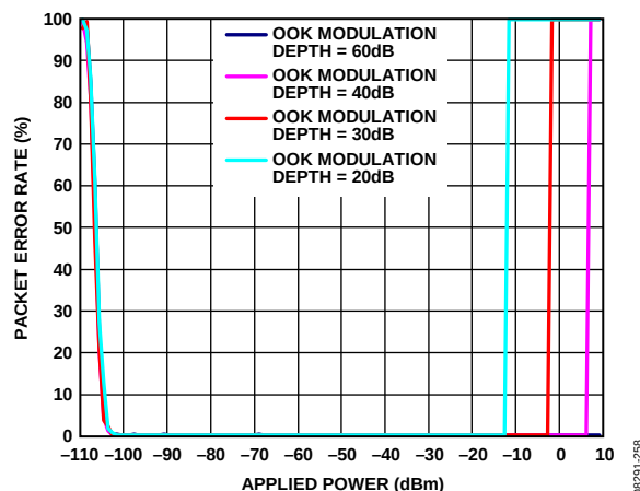
图62. OOK误包率与RF输入功率和OOK调制深度的关系： 数据速率 = 19.2 kbps (芯片速率 = 38.4 kcps, 曼彻斯特编码), IF带宽 = 100 kHz, V_{DD} = 3.6 V, 温度 = 25°C, RF频率 = 902 MHz, 前同步码长度 = 100位
