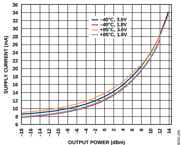
图10. 单端PA (915 MHz): 电源电流与输出功率、温度和 V_{DD} 的关系
