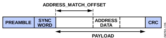
图77. 固定和可变长度包模式下的有效载荷长度
