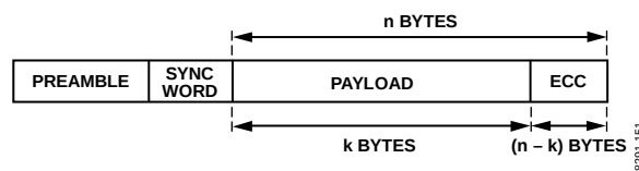
图103. 追加Reed Solomon差错校验码(ECC)的包结构
