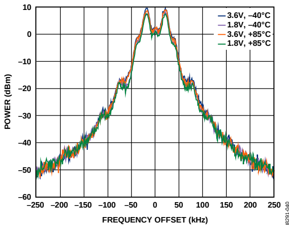
图19. 发射频谱：868 MHz、FSK、数据速率=38.4 kbps、 频率偏差=20 kHz
