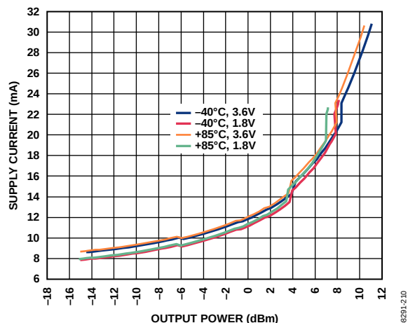
图14. 差分PA (915 MHz): 电源电流与输出功率、温度和 V_{DD} 的关系
