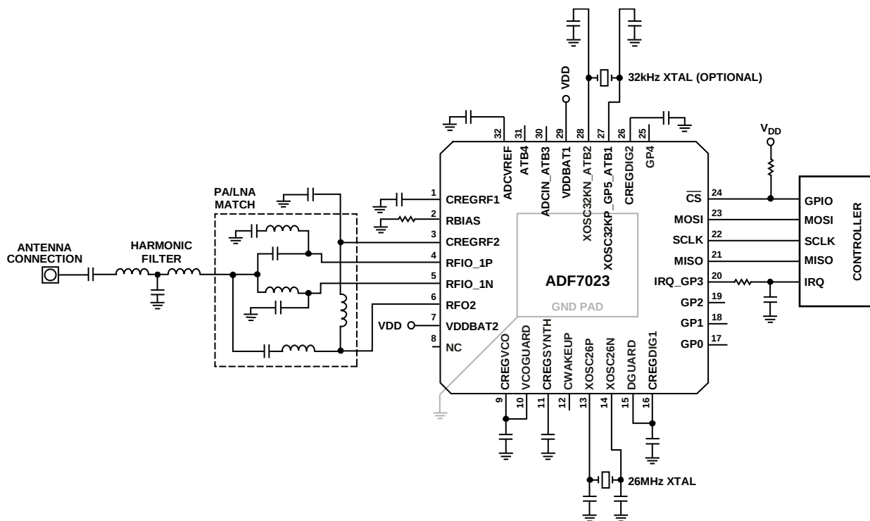
图109. ADF7023典型应用电路图
