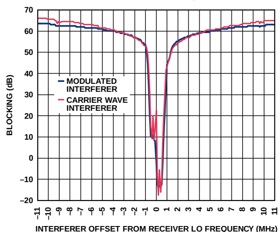
图43. 接收机宽带阻塞: 915 MHz、 数据速率 = 300 kbps
