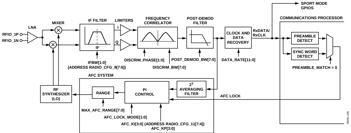
图108. 2FSK/GFSK/MSK/GMSK解调和AFC架构
