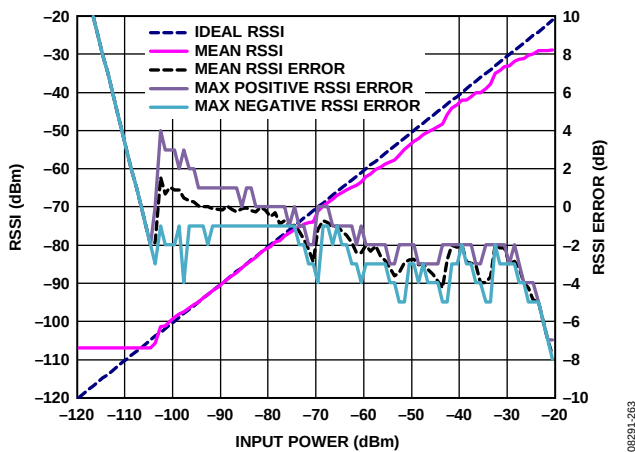
图67. RSSI（通过“自动包结束RSSI测量”）与RF输入功率的关系： 868 MHz，GFSK，数据速率 = 300 kbps，频率偏差 = 75 kHz， IF带宽 = 300 kHz，AGC_CLOCK_DIVIDE = 15， 每个输入功率电平进行100次RSSI测量
