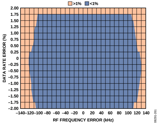
图65. AFC开启：误包率与RF频率误差和数据速率误差的关系， AFC关闭，数据速率=300 kbps，频率偏差 = 75 kHz， GFSK，AGC_LOCK_MODE = 前同步码后锁定
