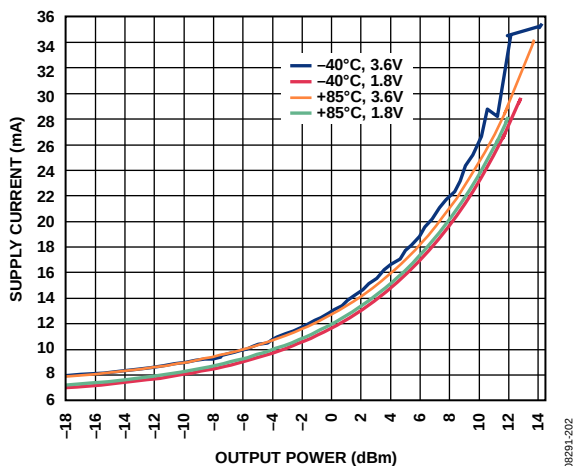
图6. 单端PA (433 MHz): 电源电流与输出功率、温度和 V_{DD} 的关系
