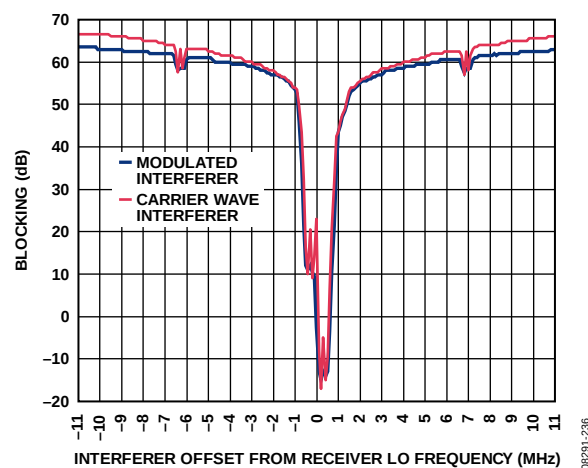
图40. 接收机宽带阻塞: 868 MHz, 数据速率 = 100 kbps
