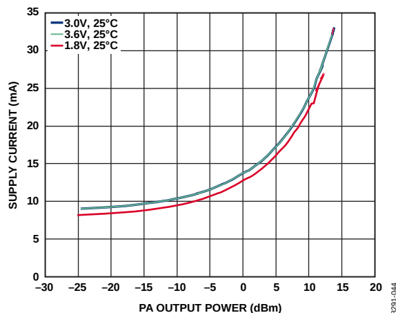
图8. 单端PA (868 MHz): 电源电流与输出功率、温度和 V_{DD} 的关系
