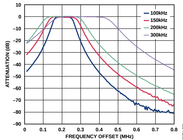
图 33. IF滤波器响应与IF带宽的关系: V_{DD} = 3.0\text{ V} , 温度 = 25^{\circ}\text{C}
