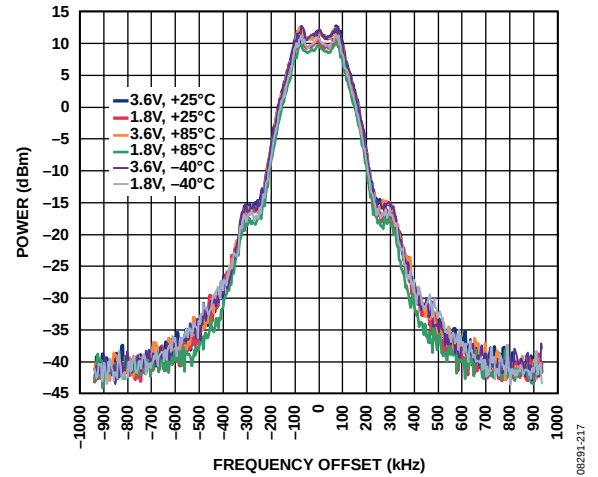
图21. 发射频谱：928 MHz、GFSK、数据速率=300 kbps、 频率偏差=75 kHz
