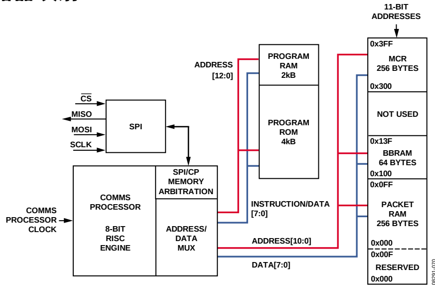
图85. ADF7023存储器映射
