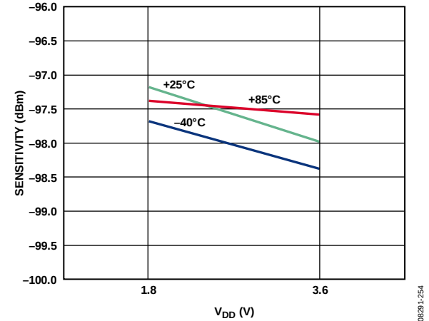
图 57. 接收机灵敏度 (误包率为 1%) 与 V_{DD} 、温度和RF频率的关系： 数据速率 = 300 kbps、GFSK、频率偏差 = 75 kHz、IF带宽 = 300 kHz
