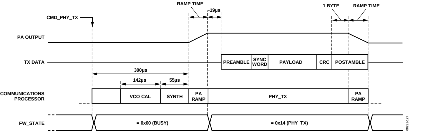
图79. 发送包时序
