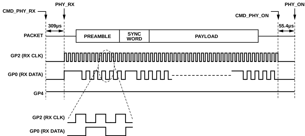
图82. Sport模式接收, DATA_MODE = 1、2且GPIO_CONFIGURE = 0xA0、0xA3、0xA6
