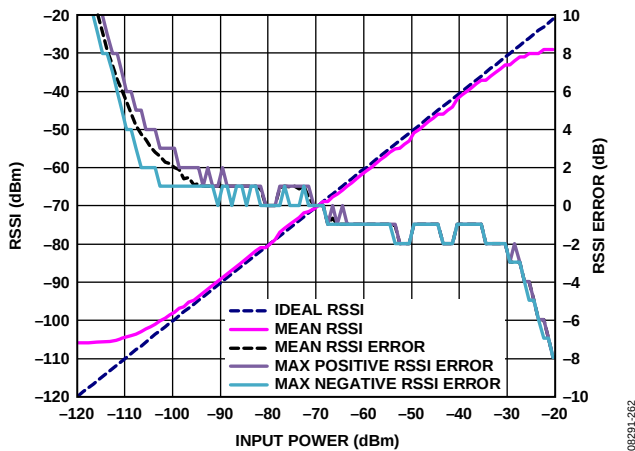
图66. RSSI（通过CMD_GET_RSSI）与RF输入功率的关系： 868 MHz，GFSK，数据速率 = 38.4 kbps，频率偏差 = 20 kHz， IF带宽 = 100 kHz，每个输入功率电平进行100次RSSI测量
