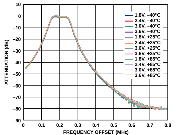
图34. IF滤波器响应与 V_{DD} 和温度的关系: 100 kHz IF滤波器带宽
