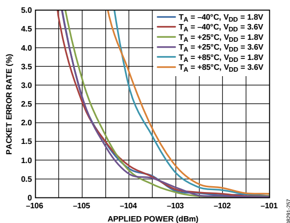
图61. OOK误包率与RF输入功率、 V_{DD} 和温度的关系：数据速率 = 19.2 kbps (芯片速率 = 38.4 kcps, 曼彻斯特编码), IF带宽 = 100 kHz, V_{DD} = 3.6 V, 温度 = 25°C, RF频率 = 902 MHz, 前同步码长度 = 100位
