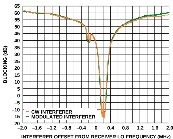
图46. 接收机带内阻塞: 915 MHz、数据速率 = 50 kbps、 IF滤波器带宽 = 100 kHz、镜像校准
