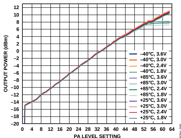
图13. 差分PA (915 MHz): 输出功率与PA_LEVEL_MCR设置、温度和 V_{DD} 的关系
