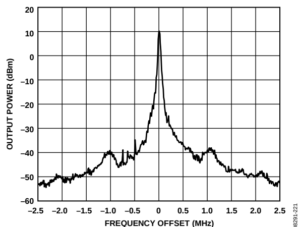
图24. OOK发射频谱: 100次扫描的最大保持、单端PA、868.95 MHz、数据速率 = 16.4 kbps (32.8 kcps曼彻斯特编码)、PA_RAMP = 1
