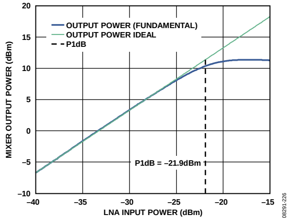
图30. LNA/混频器1 dB压缩点: V_{DD} = 3.0\text{ V} , 温度 = 25^{\circ}\text{C} , RF频率 = 915 MHz, LNA增益 = 高, 混频器增益 = 高
