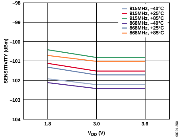
图 54. 接收机灵敏度 (比特误差率为 1E-3 ) 与 V_{DD} 、 温度和RF频率的关系：数据速率 = 300 kbps、GFSK、 频率偏差 = 75 kHz、IF带宽 = 300 kHz
