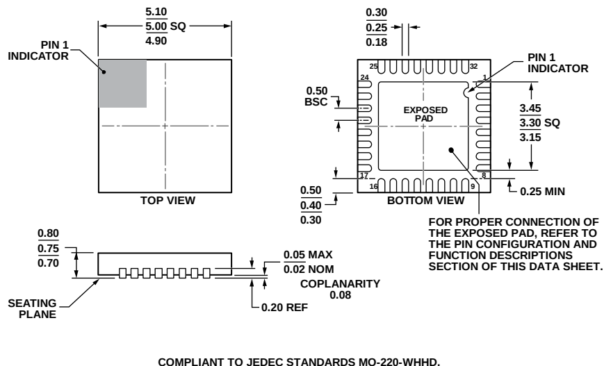
图116.32引脚引脚架构芯片级封装[LFCSP_WQ] 5 mm × 5 mm, 超薄体(CP-32-13) 图示尺寸单位: mm
