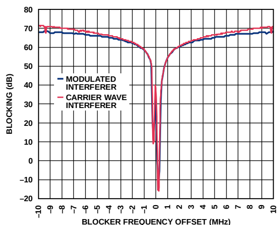
图42. 接收机宽带阻塞: 915 MHz、 数据速率 = 100 kbps
