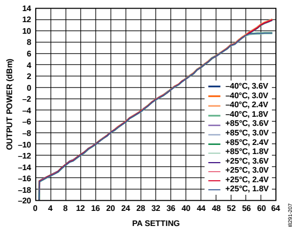
图11. 差分PA (433 MHz): 输出功率与PA_LEVEL_MCR设置、温度和 V_{DD} 的关系
