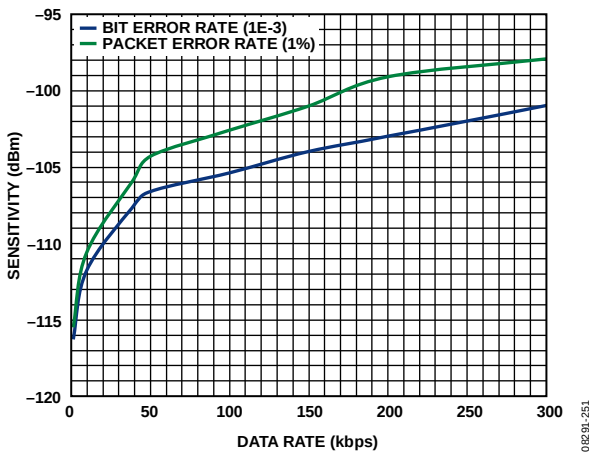
图 55. 比特误差率灵敏度 (BER = 1E-3 ) 和误包率灵敏度 (PER = 1%) 与数据速率的关系： GFSK、 V_{DD} = 3.0 V、温度 = 25°C
