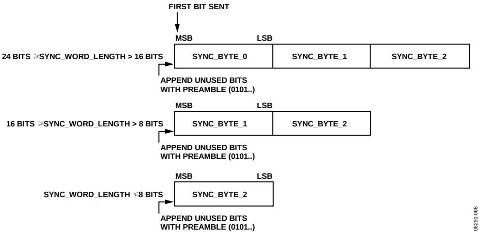
图76. 发送同步字配置
