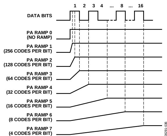
图107.不同PA_RAMP设置的PA斜坡
