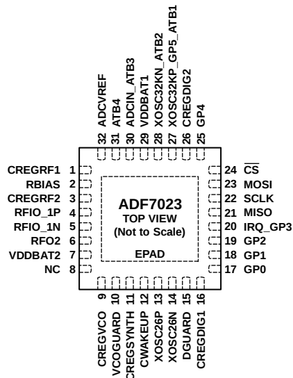
图4. 引脚配置
