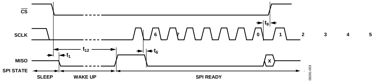
图3. PHY_SLEEP到SPI就绪状态时序( \overline{\text{CS}} 下降沿后的SPI就绪T12)
