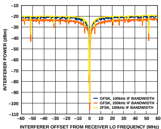
图45. 接收机宽带阻塞: 868 MHz、数据速率 = 38.4 kbps、 根据ETSI EN 300 220进行测量
