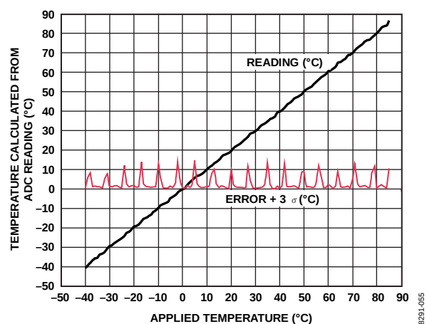
图72. 1000次温度传感器回读平均值和3 \sigma 误差与温度的关系， 3 \sigma 误差经测定为 \pm 14^{\circ}\text{C} ， V_{DD} = 3\text{ V} ，10次回读平均值精度为 \pm 4.4^{\circ}\text{C}
