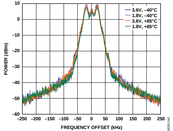
图20. 发射频谱：868 MHz、GFSK、数据速率=38.4 kbps、 频率偏差=20 kHz
