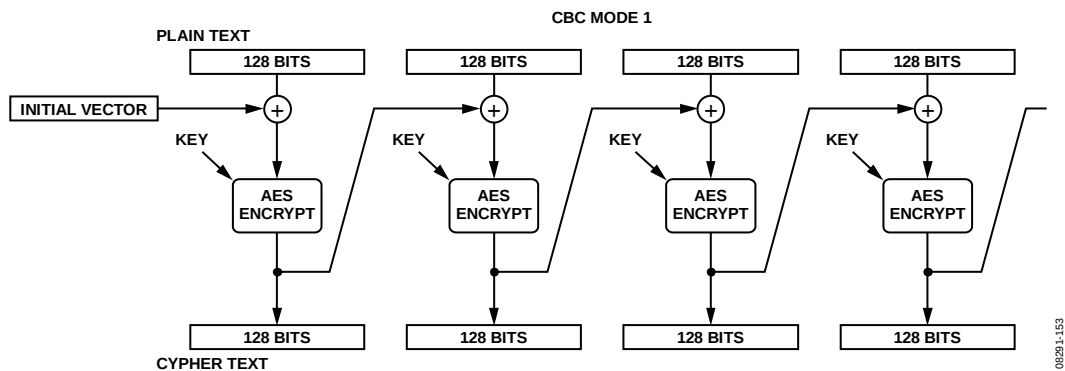
图105. CBC模式1
