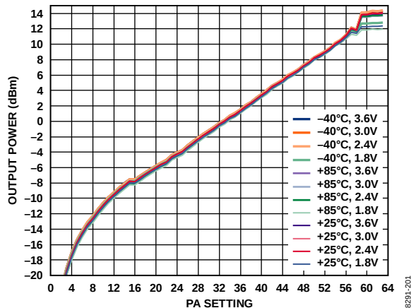
图5. 单端PA (433 MHz): 输出功率与PA_LEVEL_MCR设置、温度和 V_{DD} 的关系
