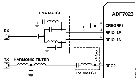
图113. 单独单端PA和LNA匹配
