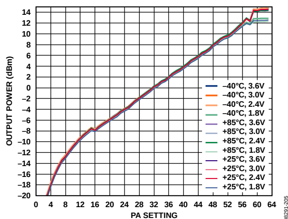
图9. 单端PA (915 MHz): 输出功率与PA_LEVEL_MCR设置、温度和 V_{DD} 的关系
