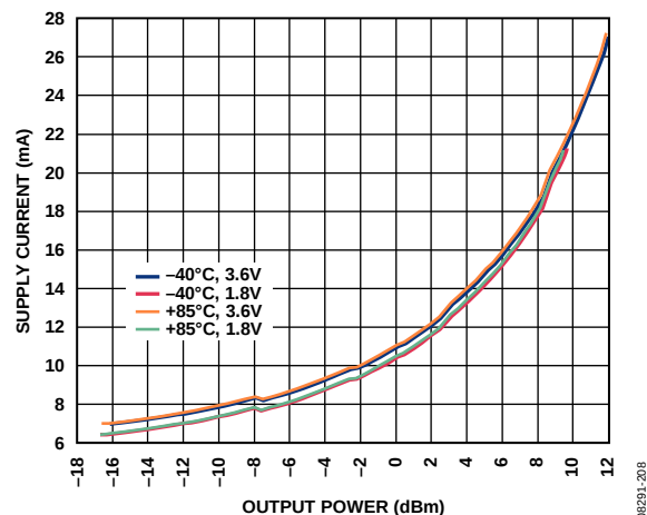
图12. 差分PA (433 MHz): 电源电流与输出功率、温度和 V_{DD} 的关系
