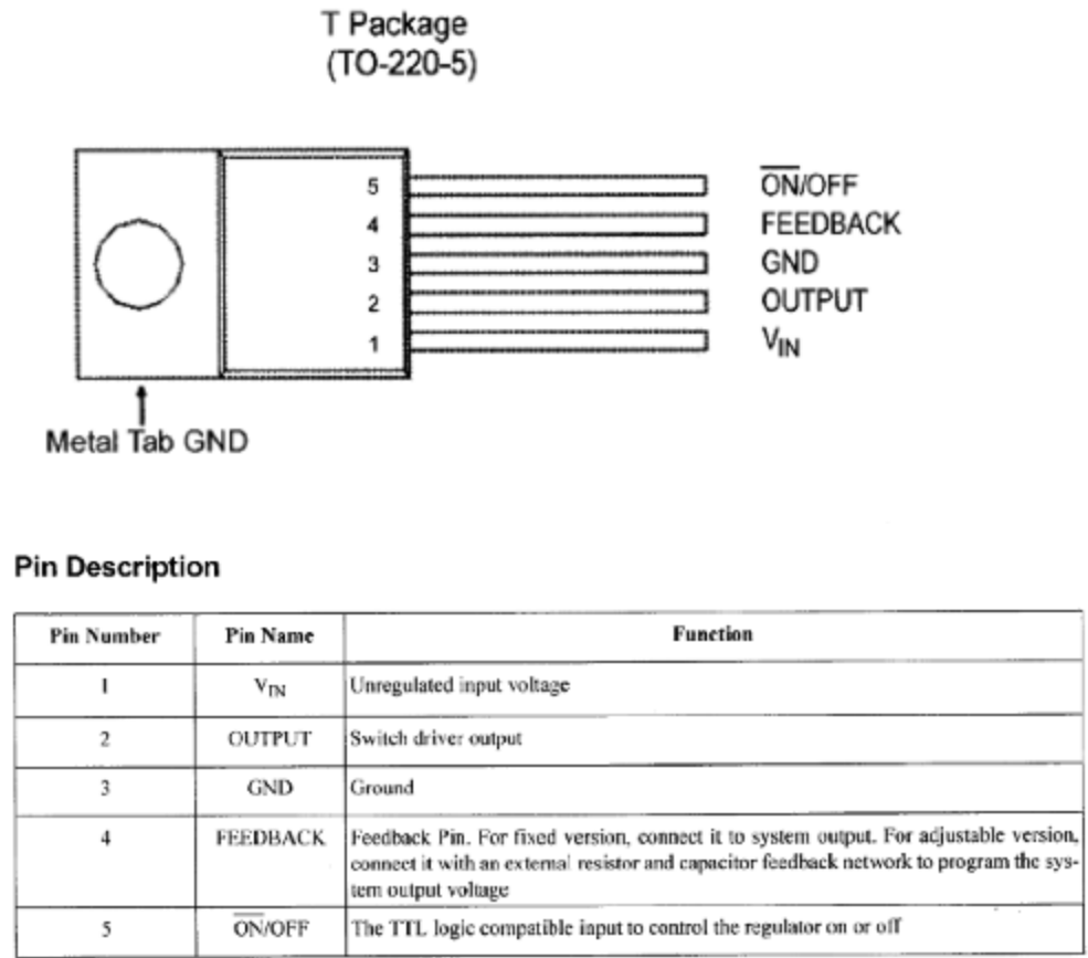
图 2 AP3003S 封装及引脚功能图
