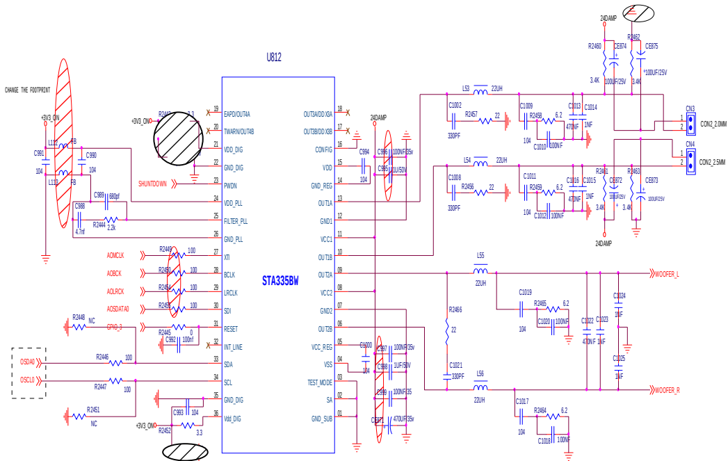
图 12 功放 STA335BW 外围电路图
