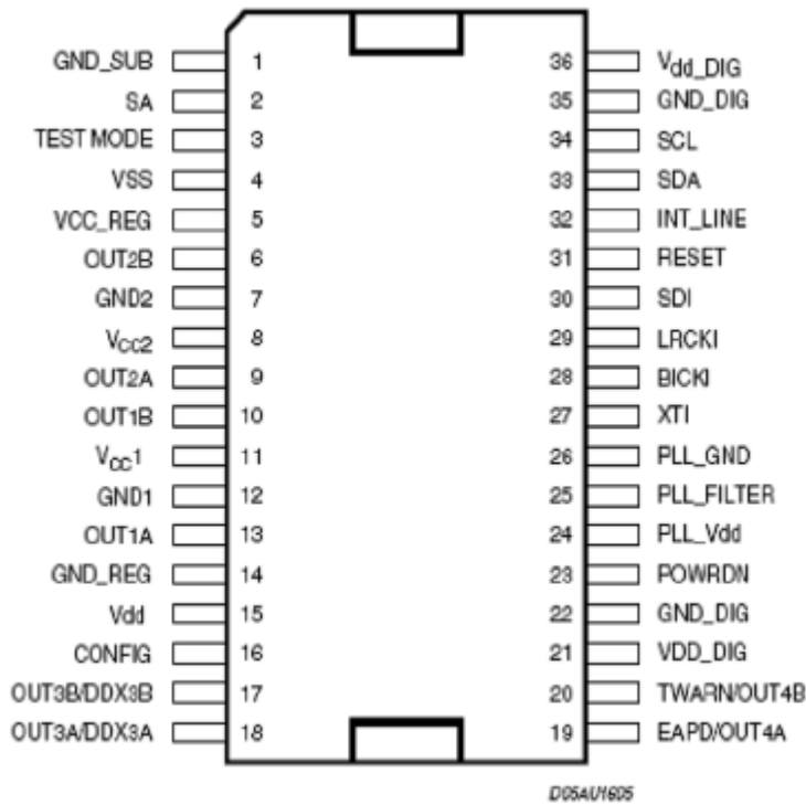
图 11 STA335BW 引脚图
