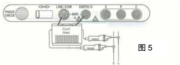
AC 电压测量
