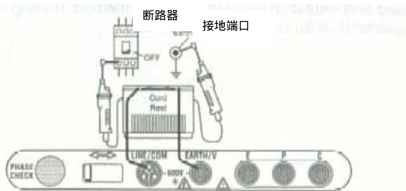
图 6 绝缘电阻测量
