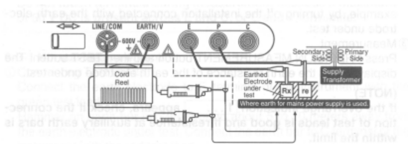
图 9 接地电阻测量（简易测量）
