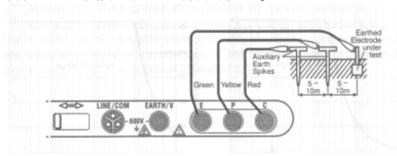
图 8 接地电阻测量（普通测量）
