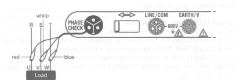
图 10 相位测量
