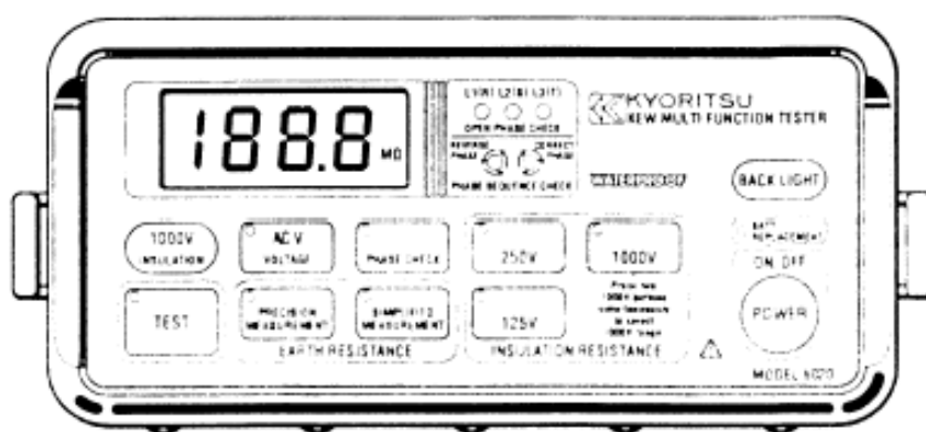
控制面板 (M-6020)
