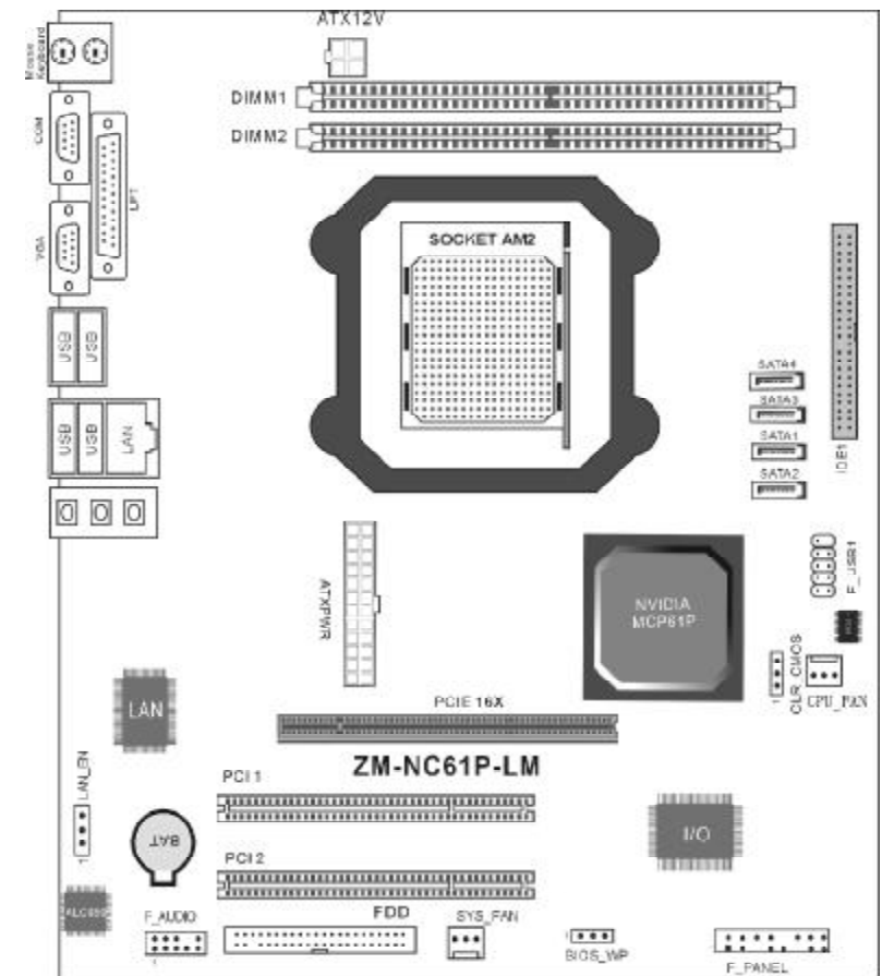
ZM-NC61P-LM (GM) 主机板布局图
