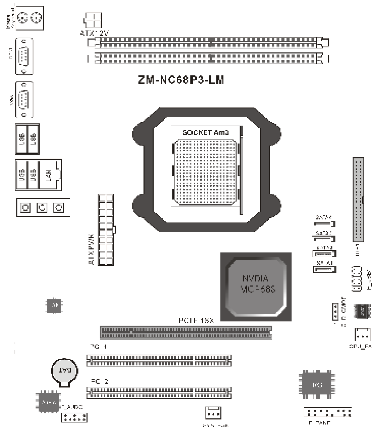
ZM-NC68P3-LM (GM) 主机板布局图
