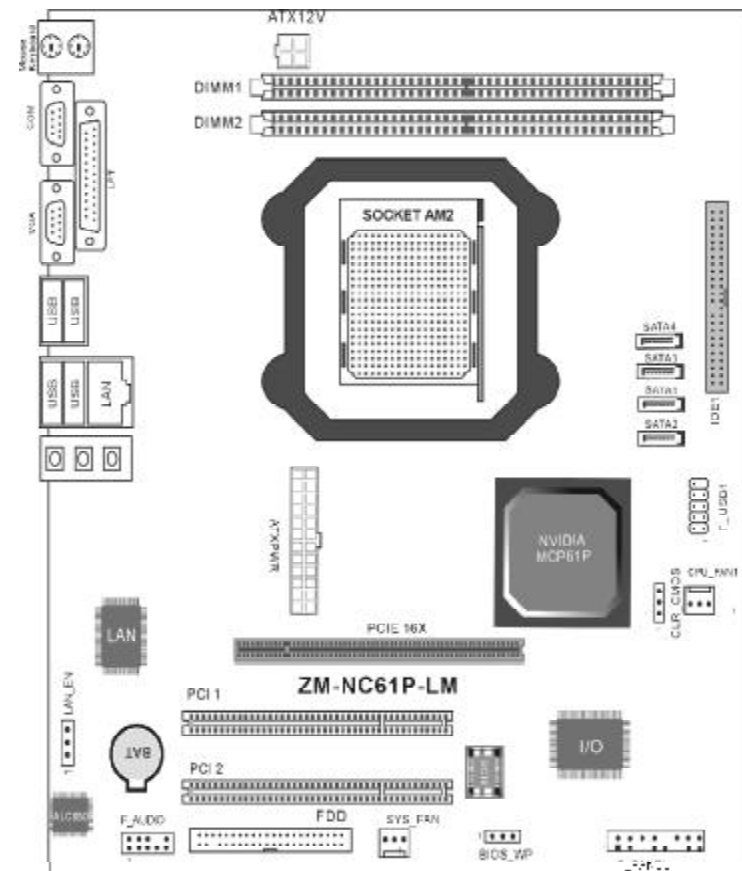
ZM-NC61P-LM (GM) 主机板布局图
