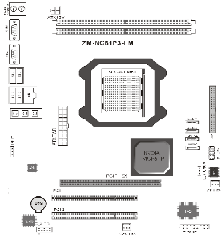
ZM-NC61P3-LM (GM) 主机板布局图
