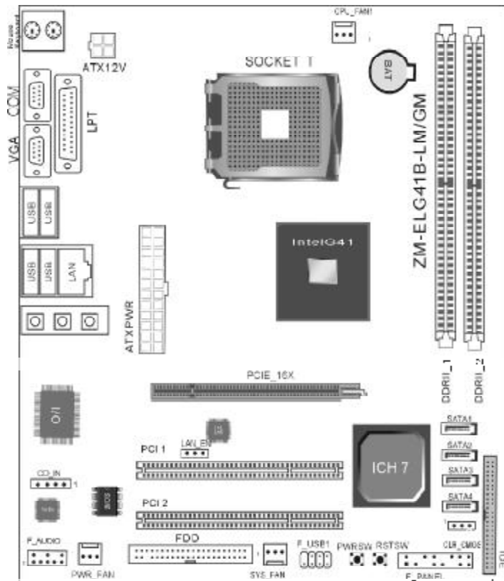
ZM-ELG41B-LM(GM)主板布局图
