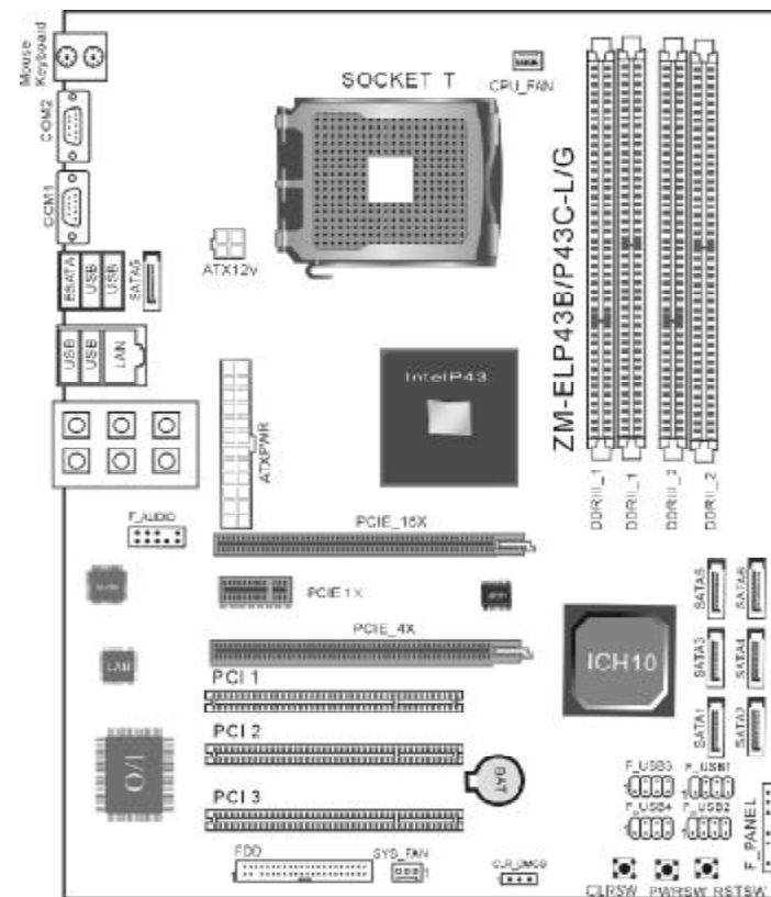
ZM-ELP43B-L(G)\ZM-ELP43C-L(G) 主板布局图
