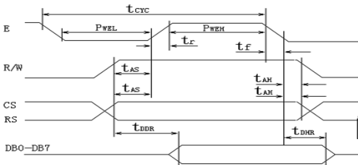
时序 2
