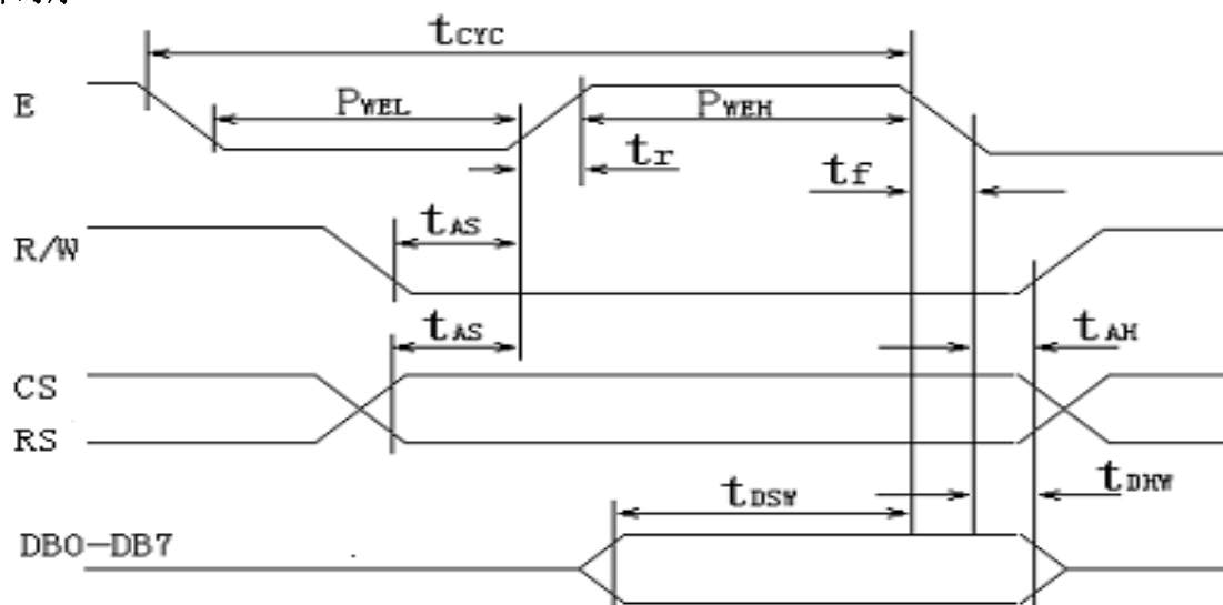
时序 1
