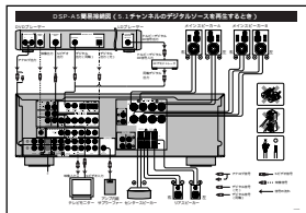
簡易接続図
