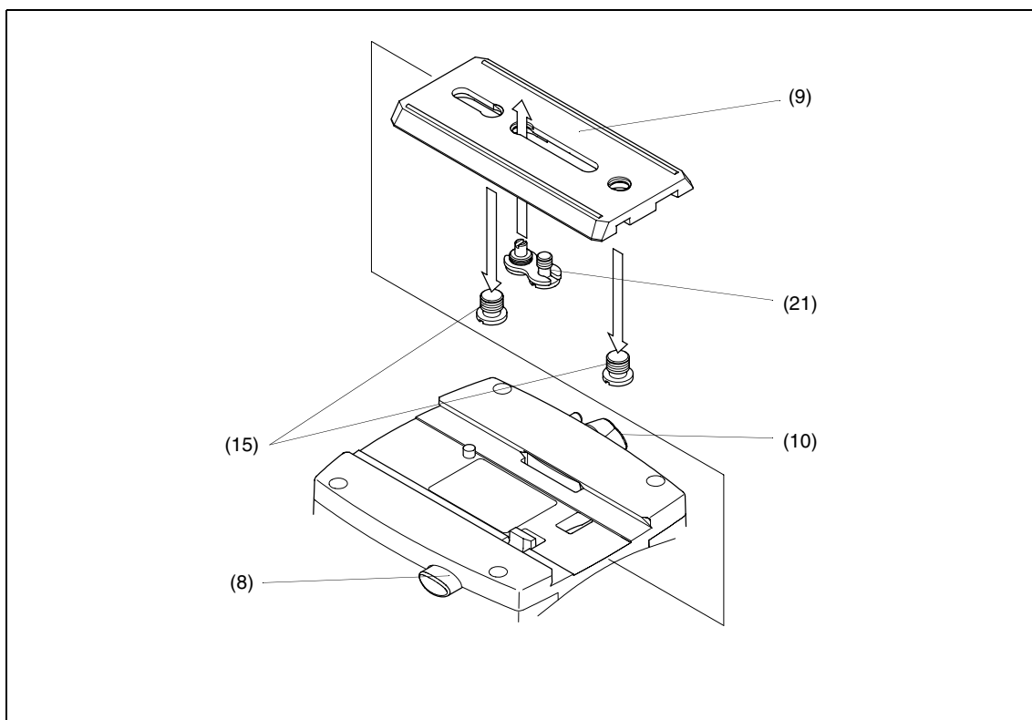
安装摄像机（VHS 适配器）
