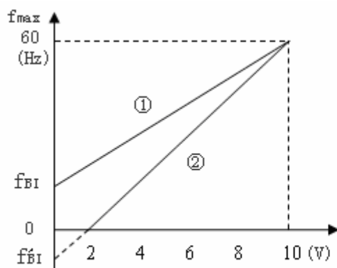
图 1 偏置频率图
