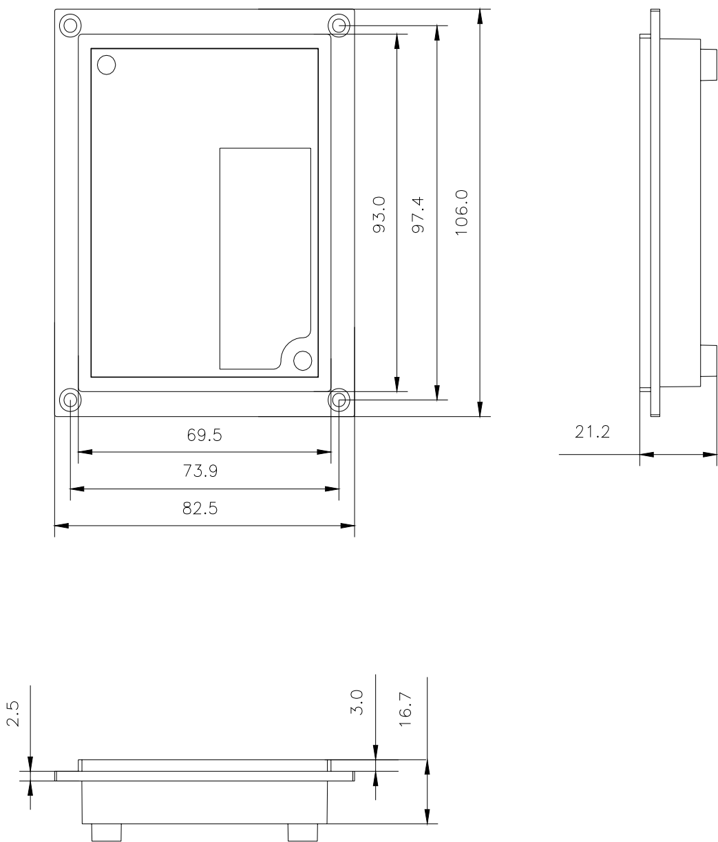
(2) Keypad 固定盒（料号：4KA82X341W01）外形尺寸：
