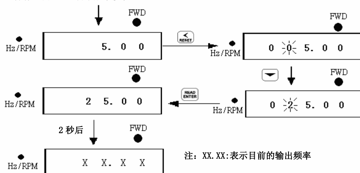
操作范例 3、运转中频率修改
