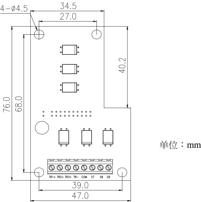
图1.1 I0扩展卡外型尺寸图
