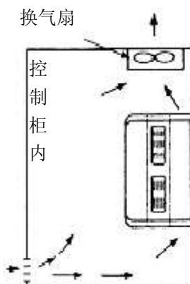
(正确的安装方式)
