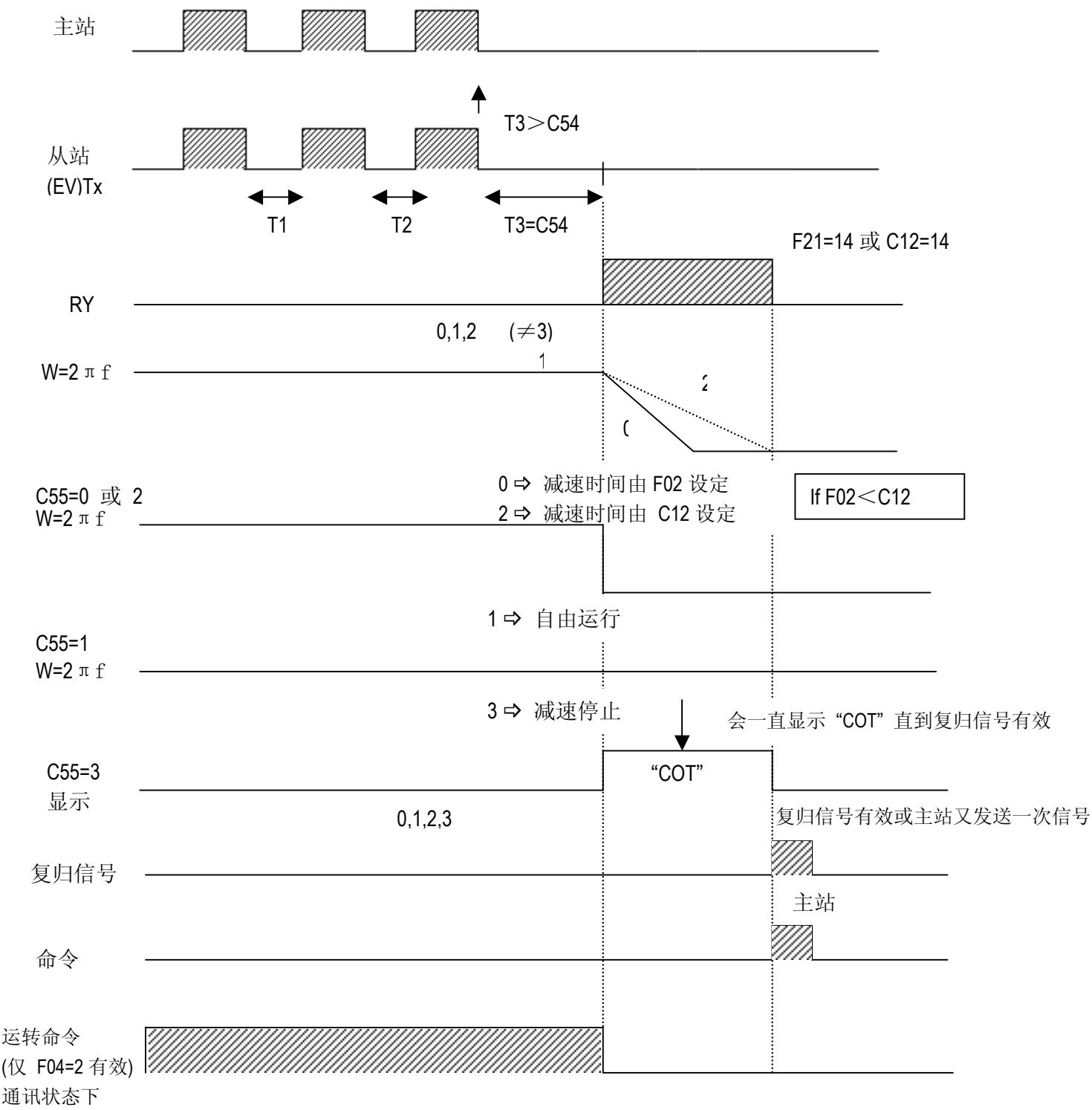
C54 / C55 通讯异常参数、通讯逾时动作时序图：
