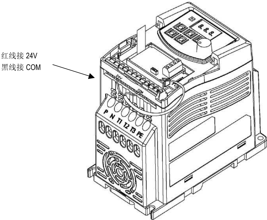
SIF-10 配线图
