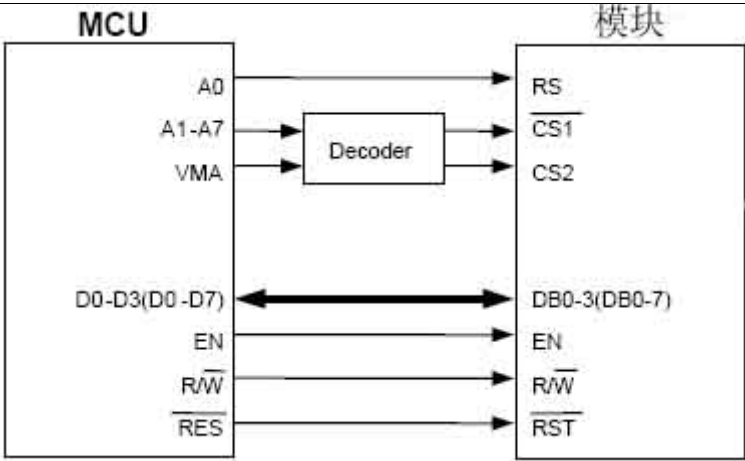
图3-3: 6800 (4/8-bit) MCU 与中文液晶显示模块的界面图
