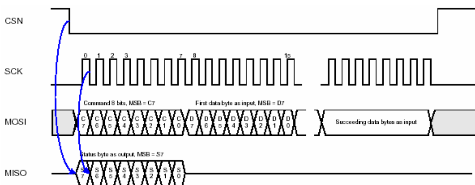
图 12: 内部 SPI 写操作时序。
