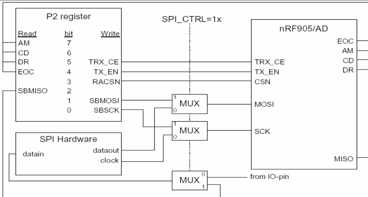
图 4 无线收发器接口
