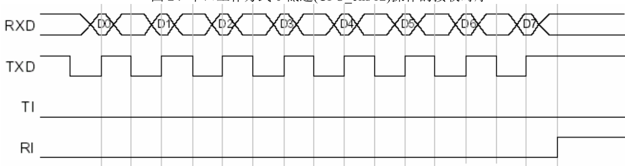
图 25 串口工作方式 0 高速(CPU_clk/4)操作的接收时序
