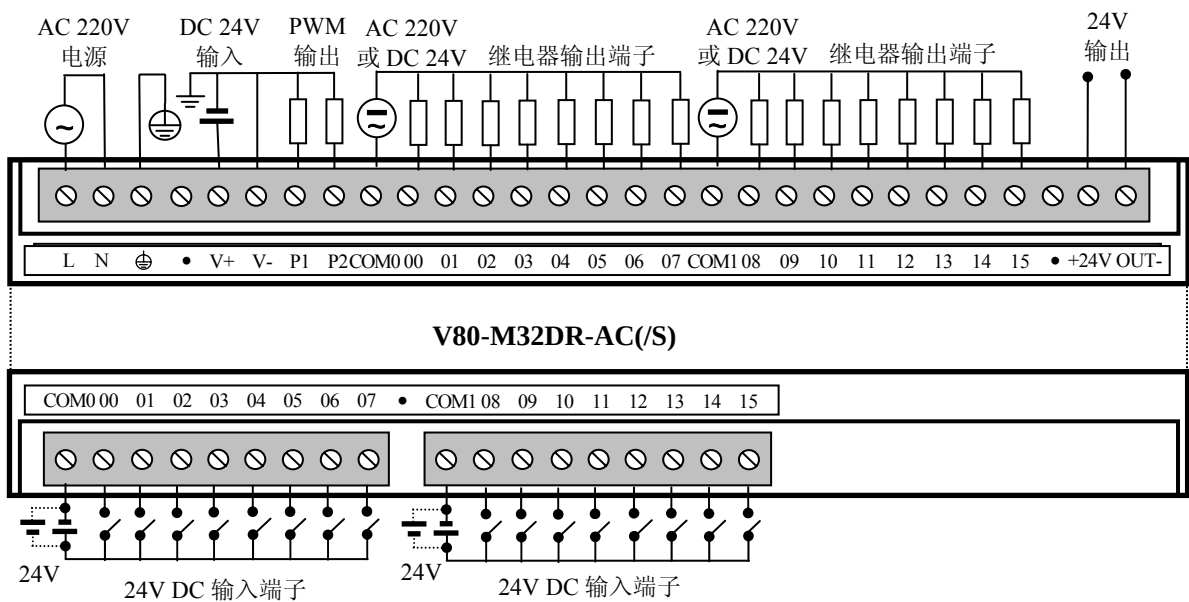
图 2.11 M32DR-AC(/S)的 I/O 端子连接图
