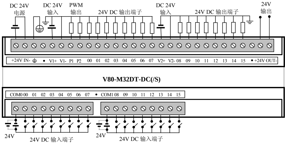
图 2.14 M32DT-DC(/S)的 I/O 端子连接图
