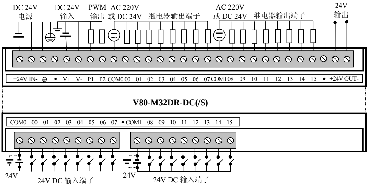
图 2.12 M32DR-DC(/S)的 I/O 端子连接图
