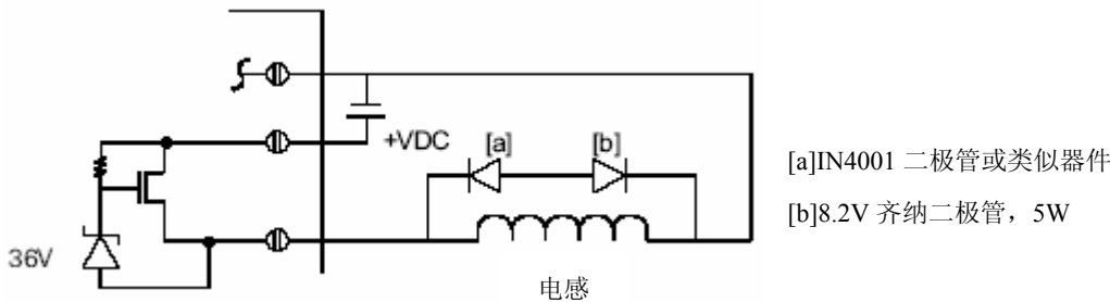
图 3.11 直流晶体管输出的齐纳二极管抑制
