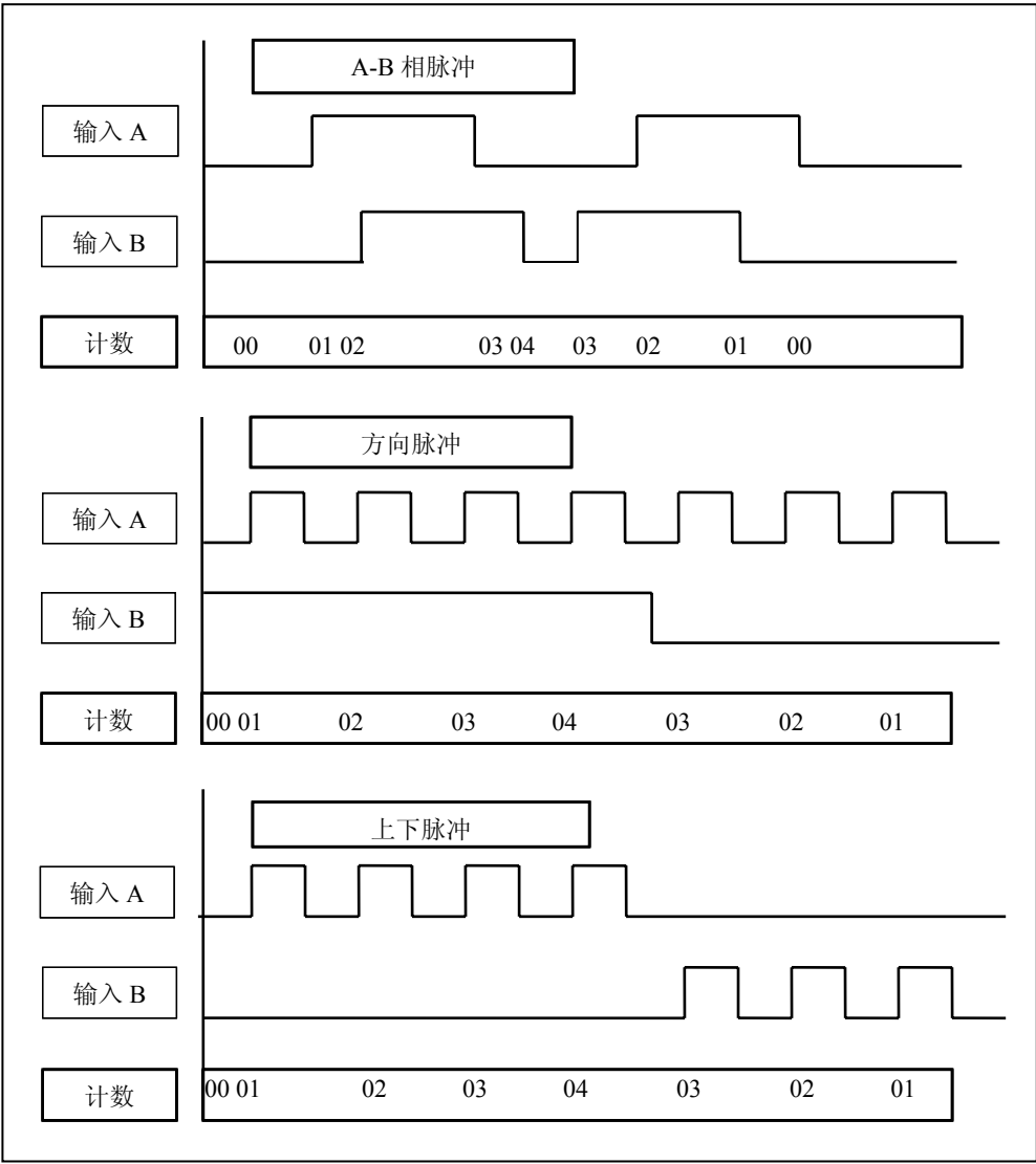
图 2.15 CPU 本体高速计数器的输入类型
