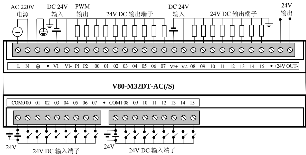
图 2.13 M32DT-AC(/S)的 I/O 端子连接图
