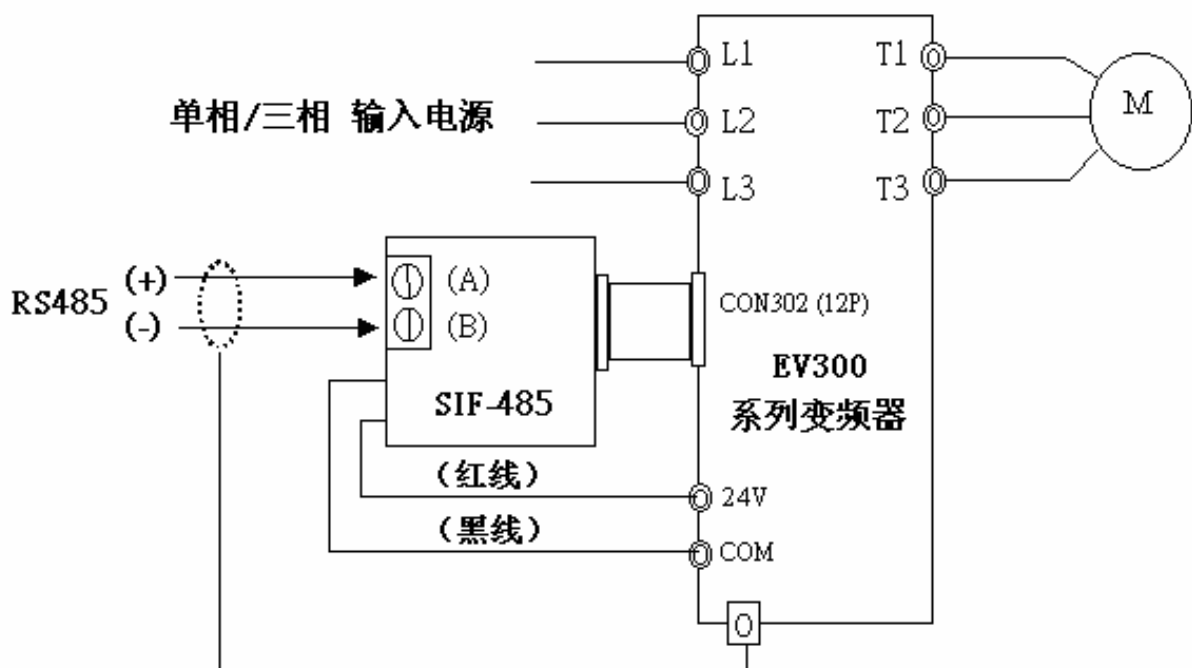
SIF-485 配线图：
