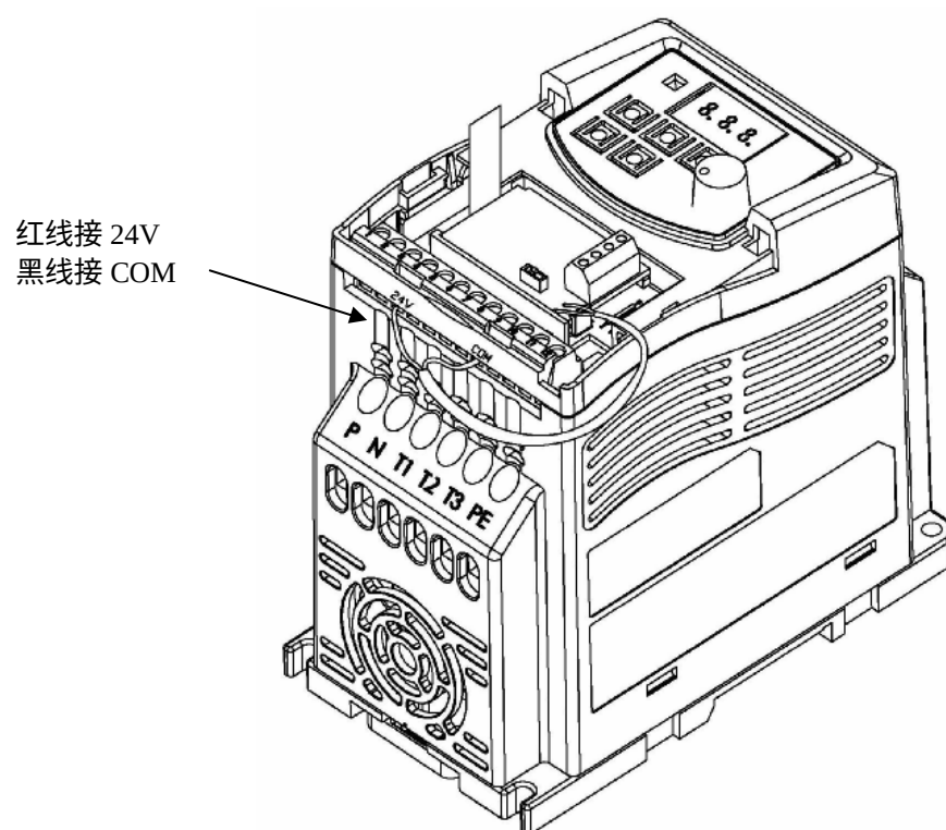
SIF-IO 配线图
