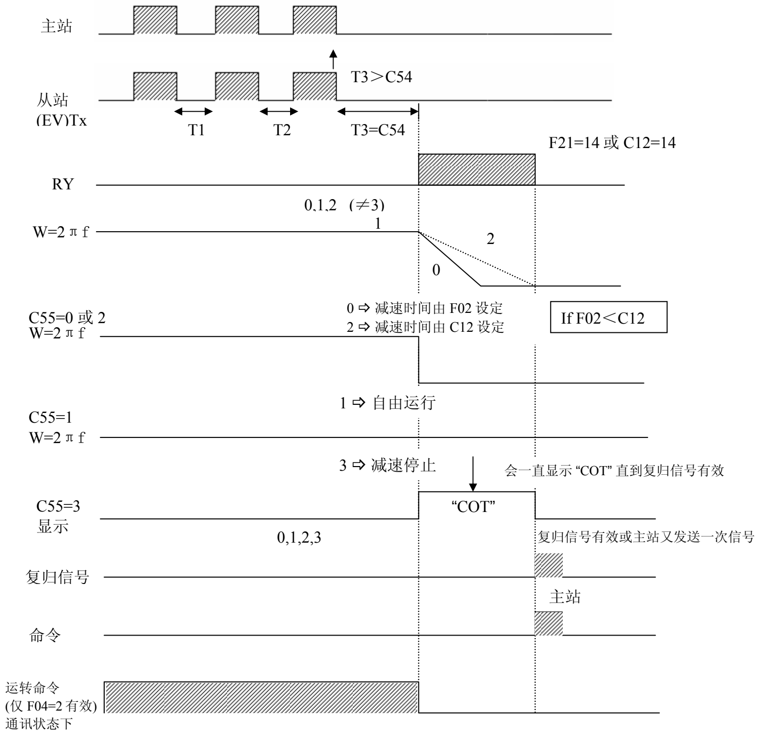
C54 / C55 通讯异常参数、通讯逾时动作时序图：
