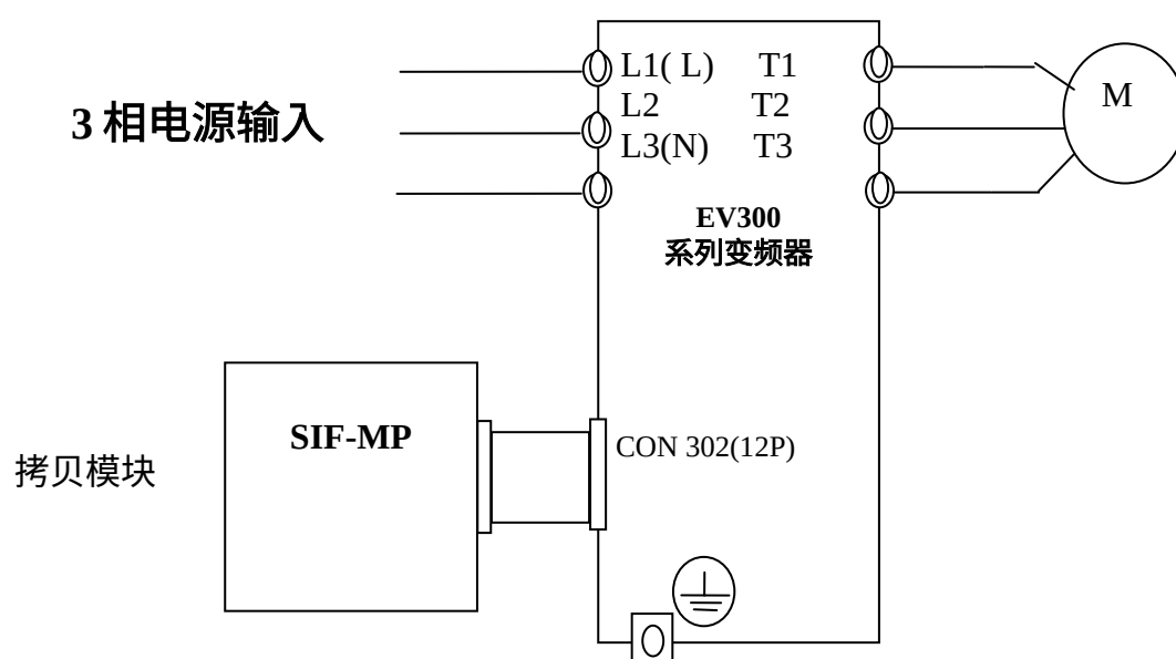
SIF-MP 配线图
