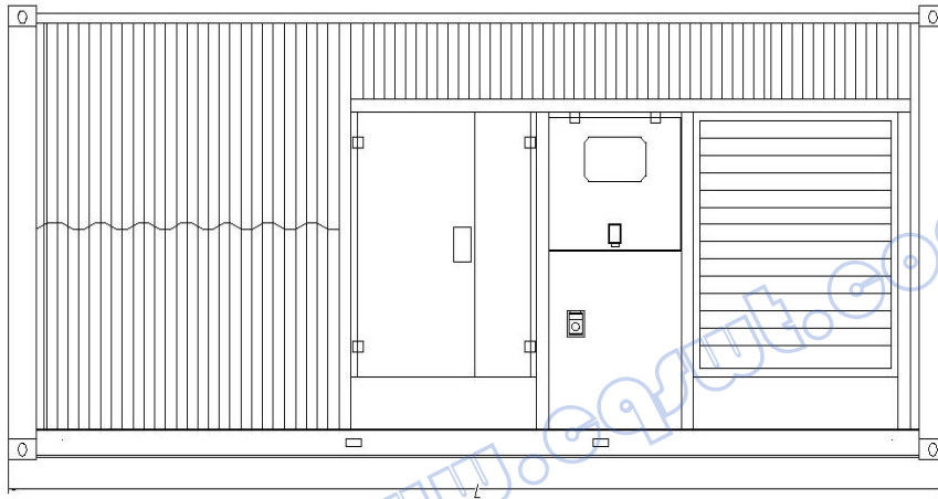
静音型： 外形尺寸 L \times W \times H (MM)=6058×2434×2591 重量 (kg)=10150 *重量数据为近似值。
