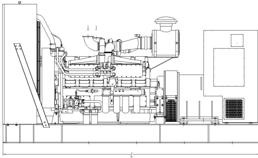
开式机组： 外形尺寸 L \times W \times H (MM)=4490×1630×2430 重量 (kg)=7800 *重量数据为近似值。
