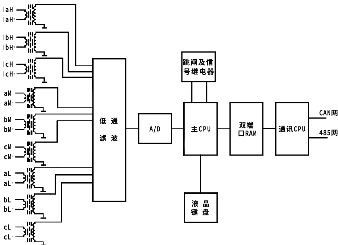
图 3.1 UT-9931C 变压器主保护装置硬件框图
