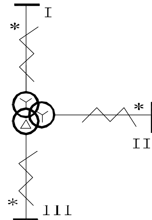
图 3.4 电流互感器连接极性
