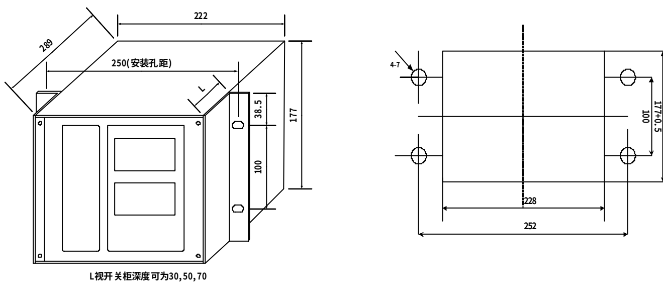
机箱外形尺寸及安装开孔尺寸（二）
