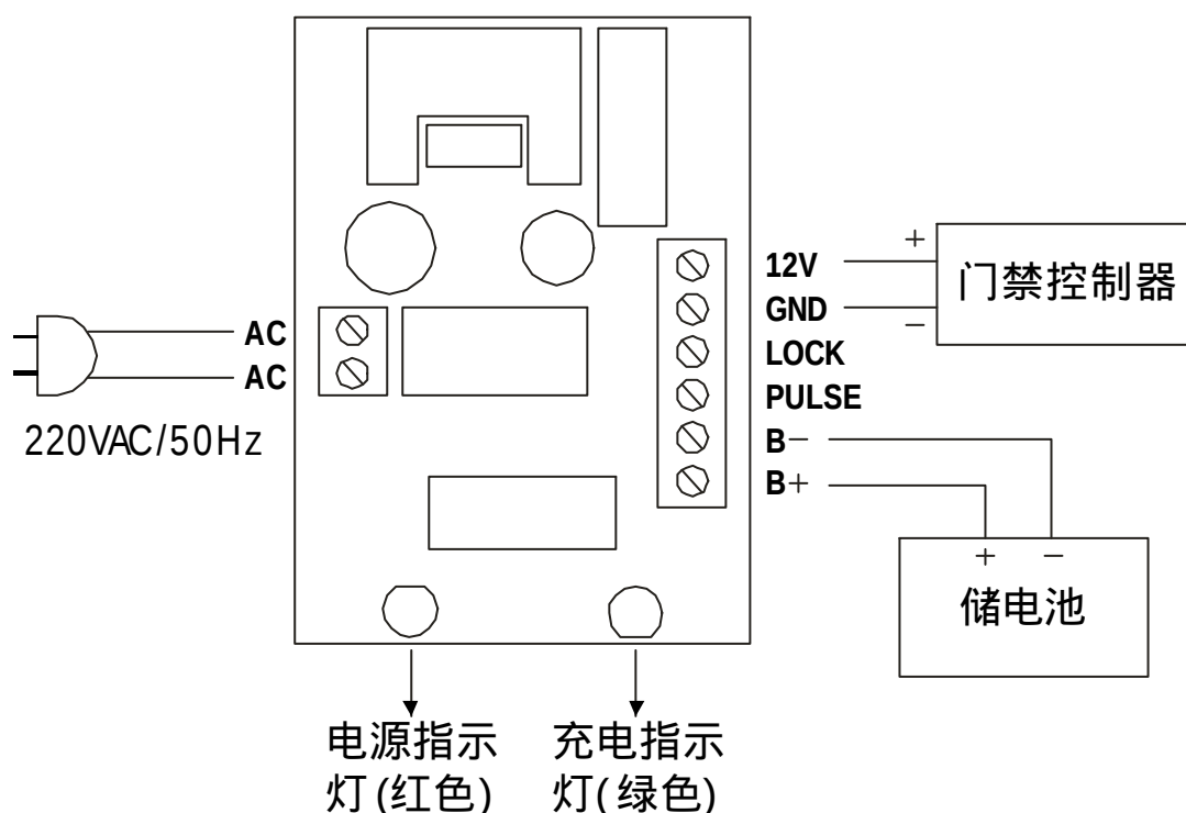
UPS12V3A 电源接线示意图
