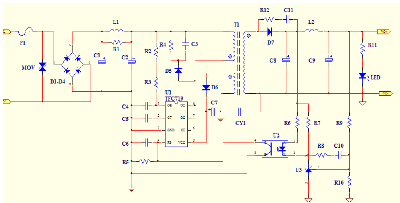
图10. 典型应用电路
