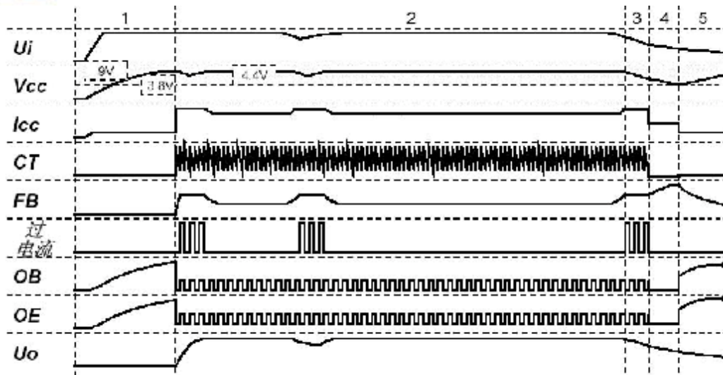
图3. 全局波形图
