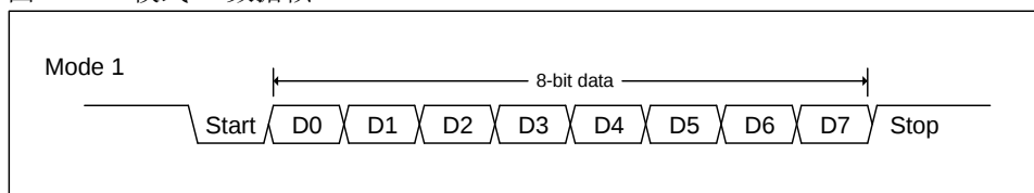
图 122-1 模式 1 数据帧
