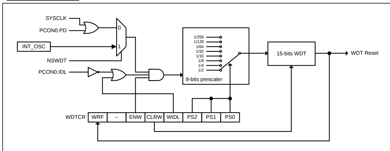
图 18-1. WDT 方框图
