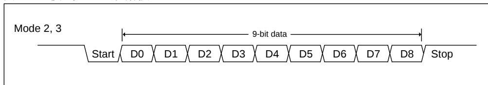
图 12-2 模式 2、3 数据帧
