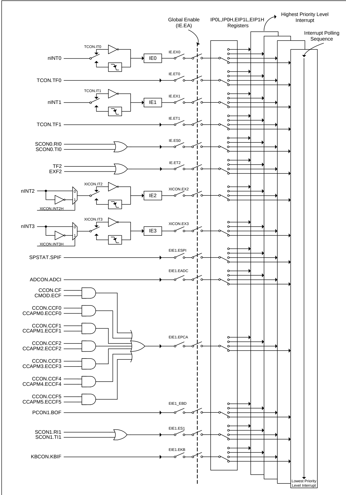
图 10-1 中断系统
