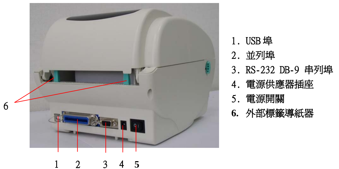
圖二 後視圖
