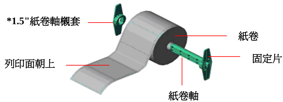
圖四 標籤安裝一
