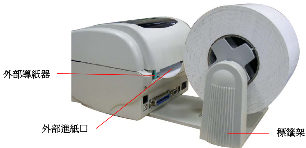
圖十一 外部籤架安裝二
