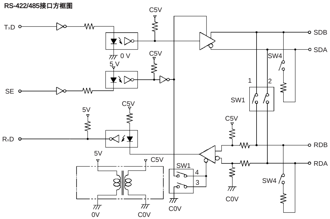
2.RS-422/RS-485 开关 (SW1) 选择 RS-422 或 RS-485 通信。
