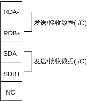
RS-485 连接时的端子图
