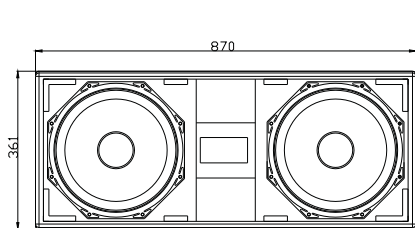
正视Front
