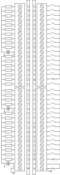
EM 223 24V DC 数字组合 32 输入/32 继电器输出 (6ES 7 223-1PM22-0XA8)
