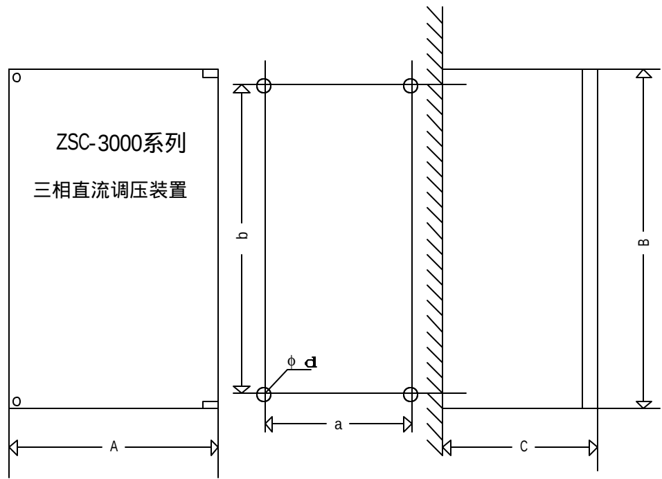
附 图 一 装置外形及安装尺寸
