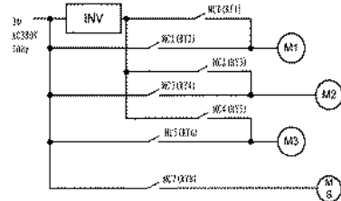
图 5 .Cd160=11,12 时
