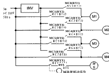
图 6 .Cd160=13,14 时
