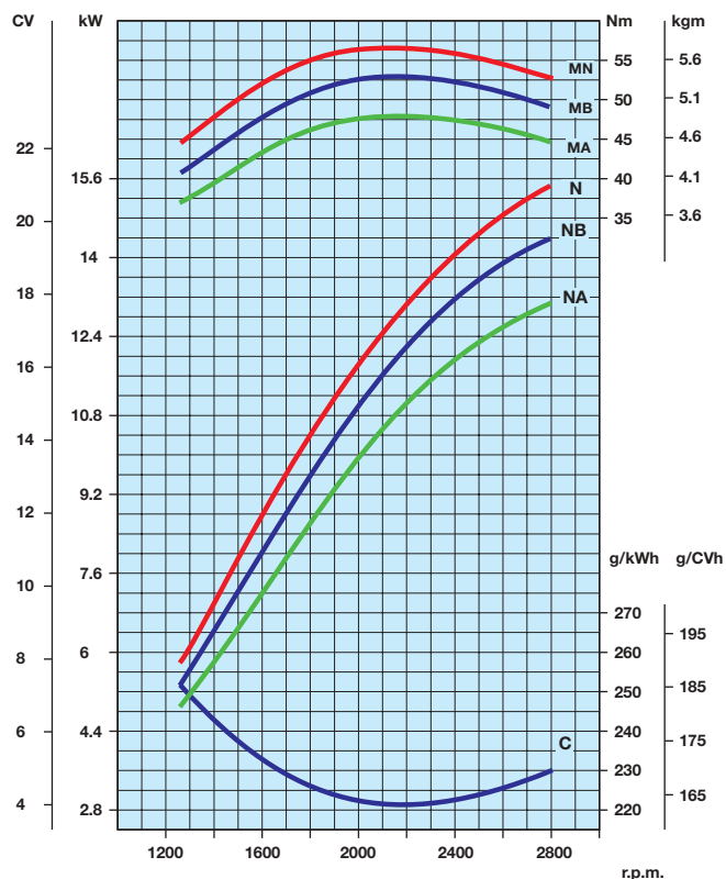
12LD 477/2 B2 @ 2800 r.p.m. ▲
