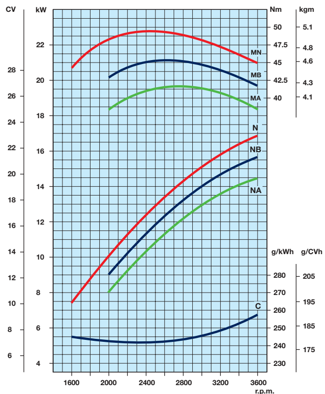
12LD 477/2 @ 3600 r.p.m.
