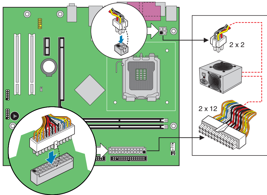
图 22. 连接 2 x 12 电源系统电缆
