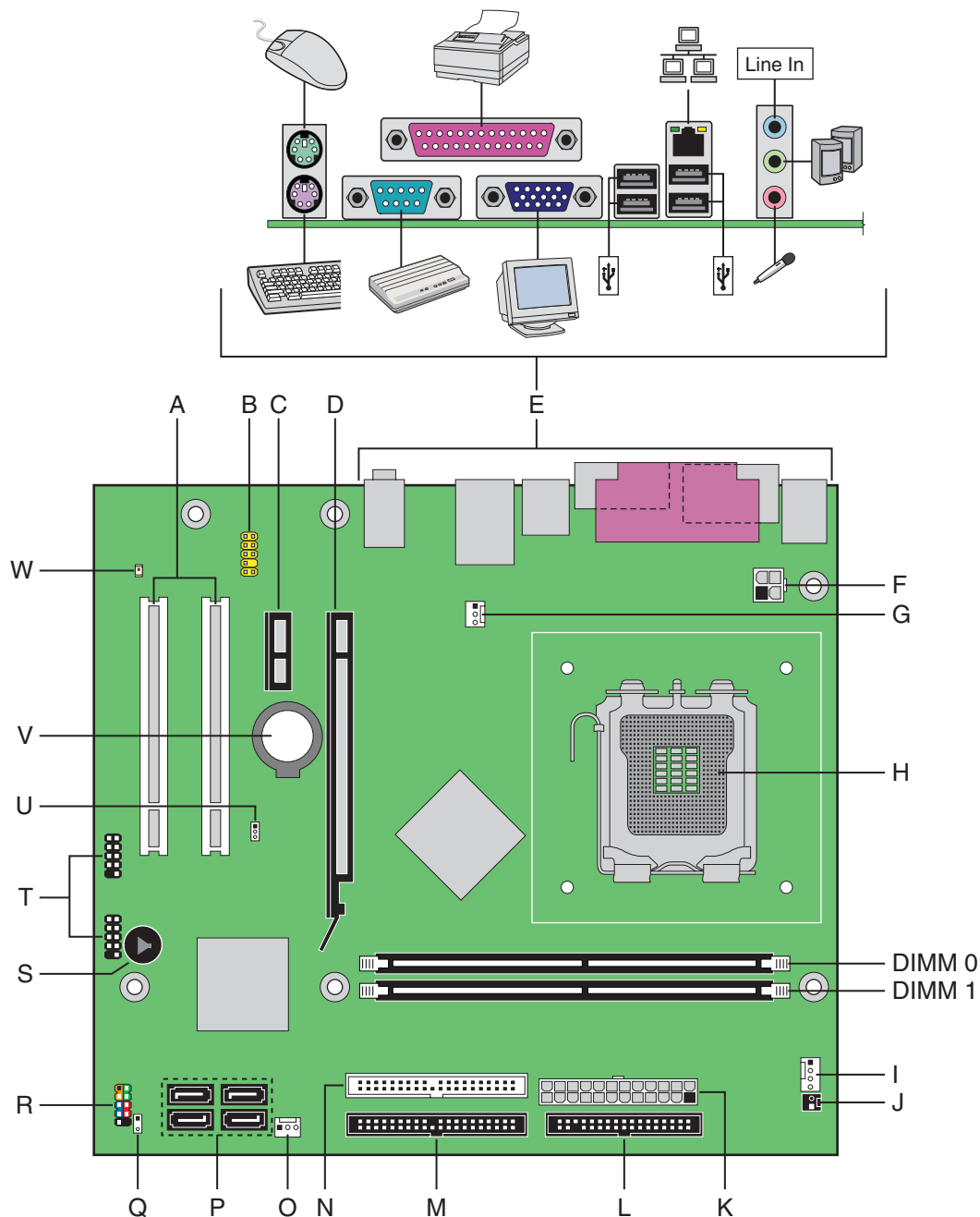
图 1. 英特尔台式机主板 D102GGC2 组件
