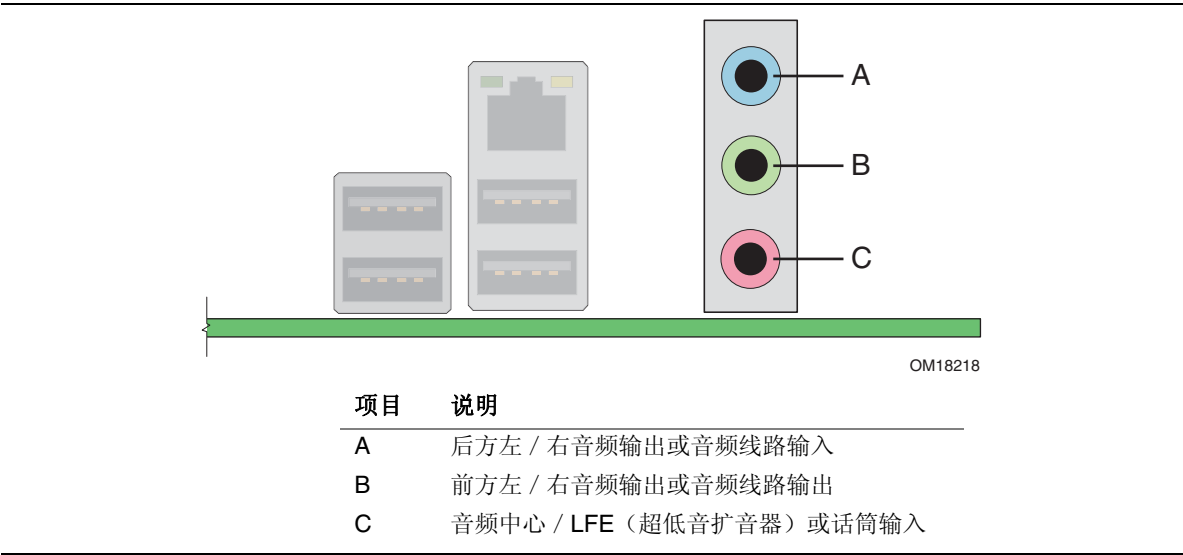
图 20. 灵活 6 声道音频系统背面板音频连接器
