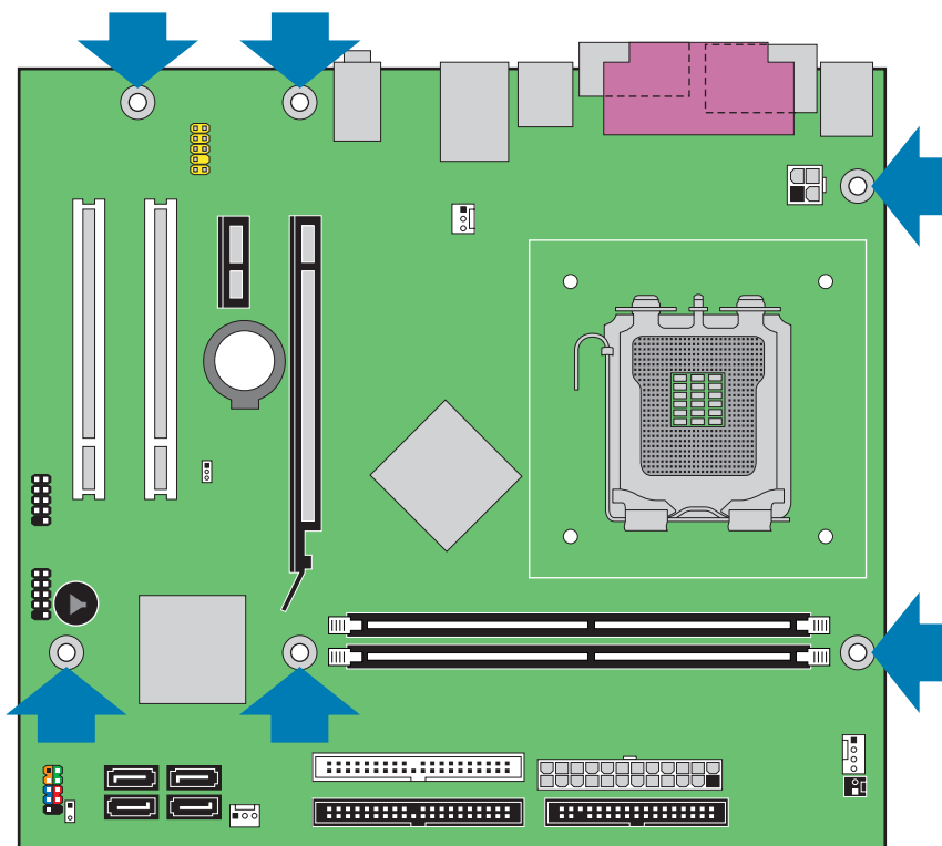
图 5. 台式机主板 D102GGC2 安装螺丝孔位置
