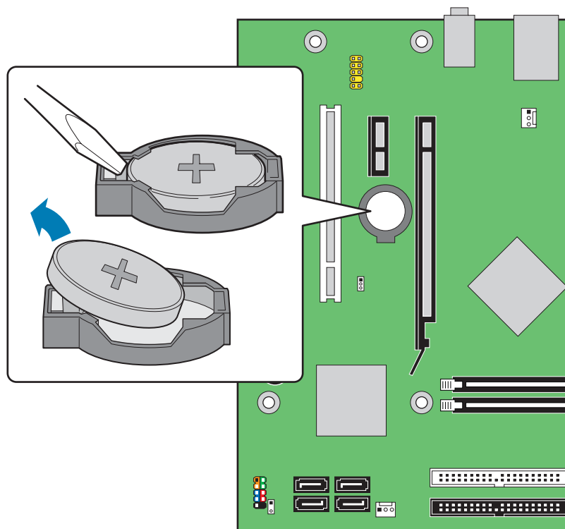
图 25. 拆卸电池
