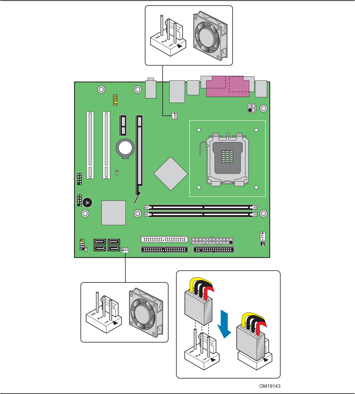
图 21. 机箱风扇接头连接器位置
