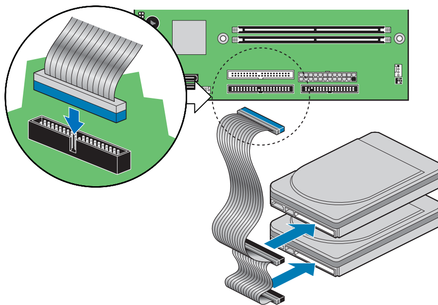
图 17. 连接 IDE 电缆
