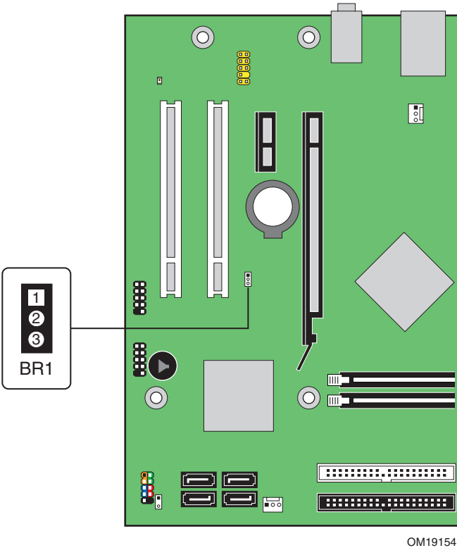
图 24. BIOS 配置跳线块位置
