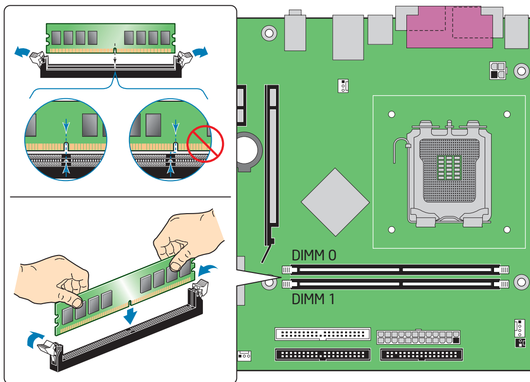
图 14. 安装 DIMM
