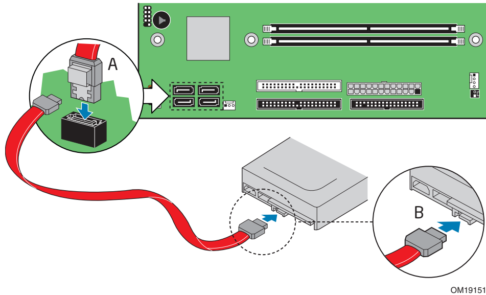
图 18. 连接串行 ATA 电缆
