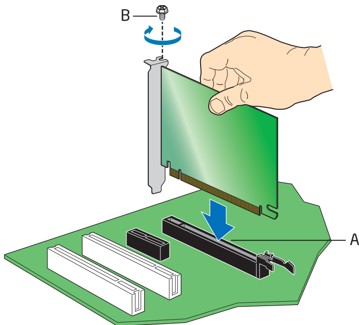
图 15. 安装 PCI Express x16 卡
