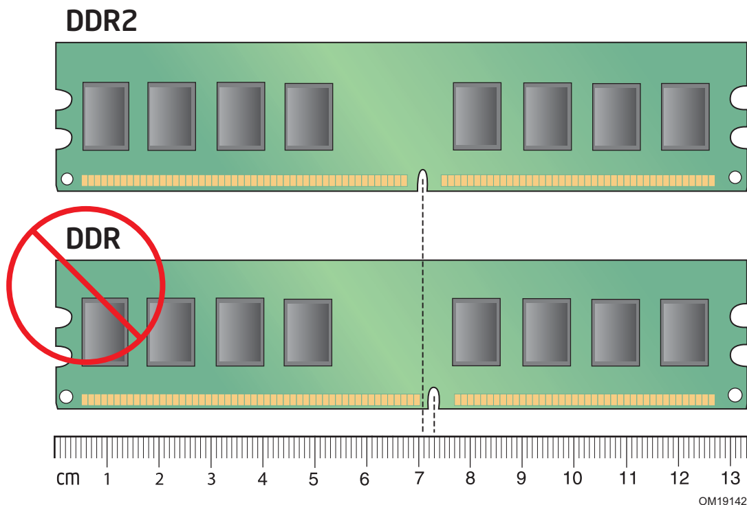
图 13. 使用 DDR DIMM
