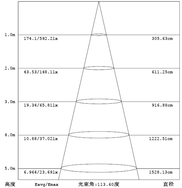
AL-L18-BE（透明面罩）照度分布图
