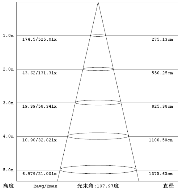
AL-L18-BE（扩散面罩）照度分布图
