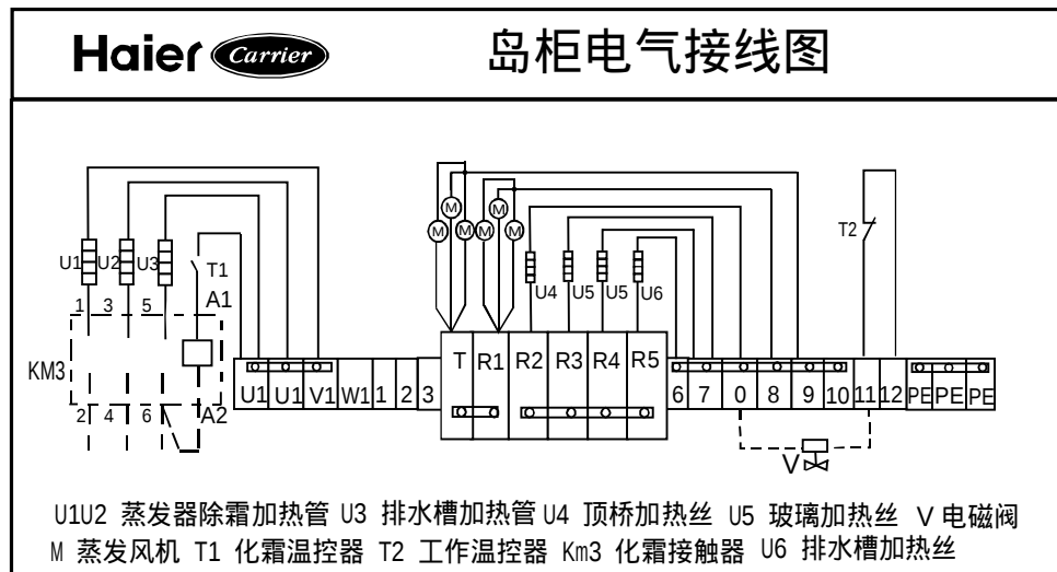
卡西娅系列岛柜接线图
