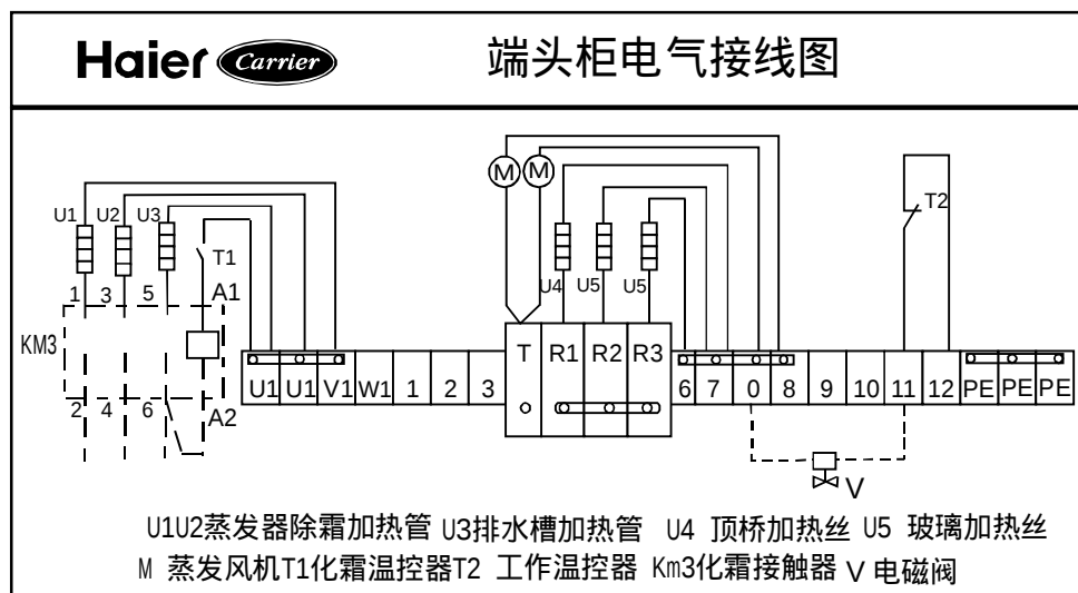
卡西娅系列端头柜接线图
