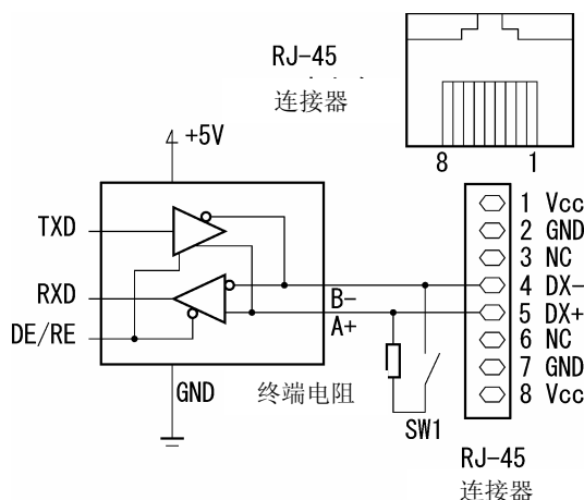
图 2.5 RJ-45 连接器的引脚排列
