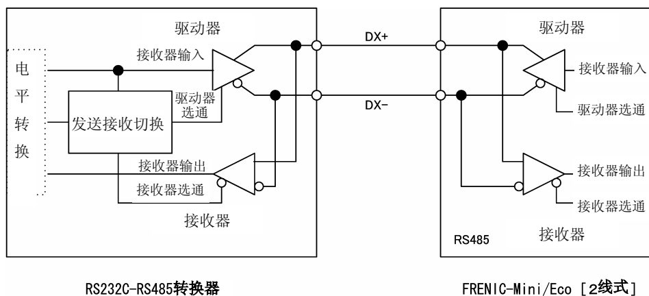
图 2.8 通信电平转换
