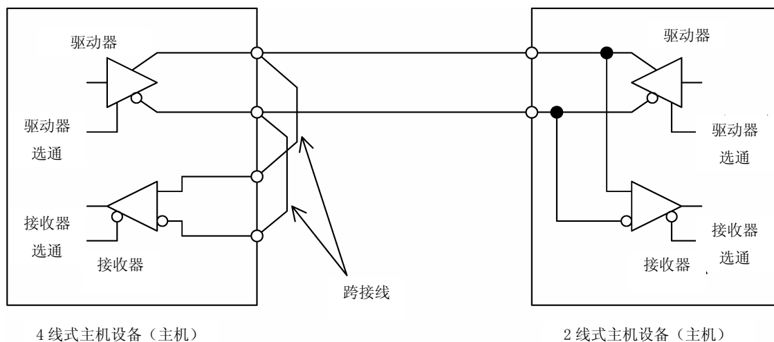
图 2.7 和 4 线式主机设备的连接
