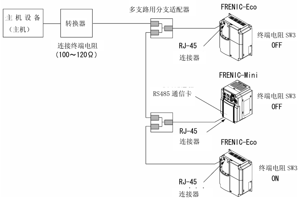
图 2.3 多支路连接图（RJ-45 连接器连接）
