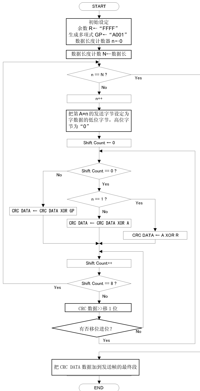
图 3.1 CRC 的算法
