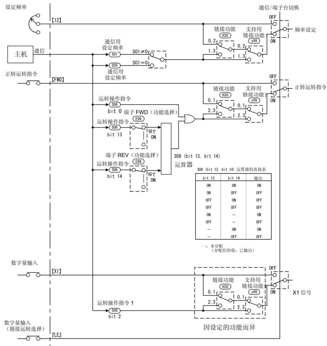
图 2.9 通信的指令系统框图
