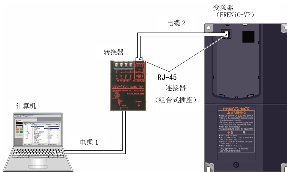
图 2.2 和计算机的连接
