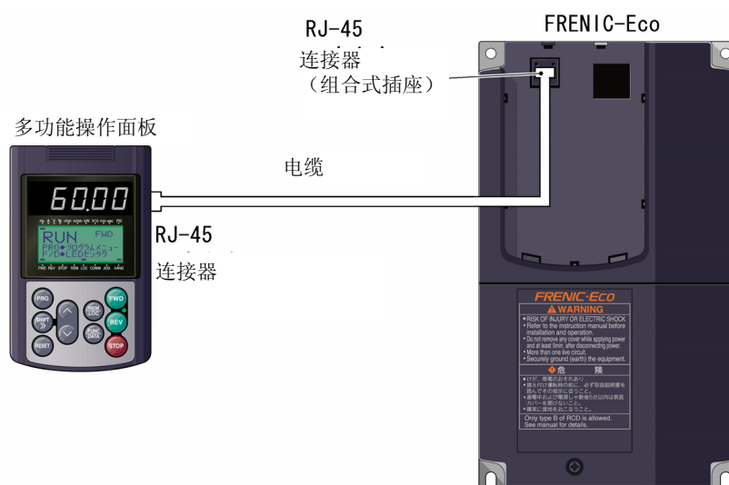
图 2.1 和操作面板的连接
