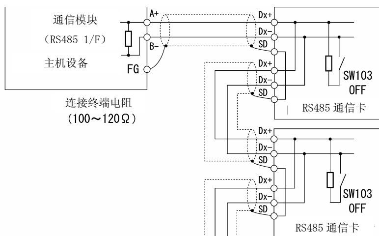
图 2.4 多支路连接图（端子台连接）
