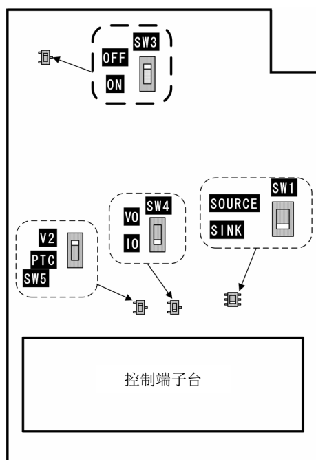
(b) 控制电路板 (FRENiC-VP 主体)
