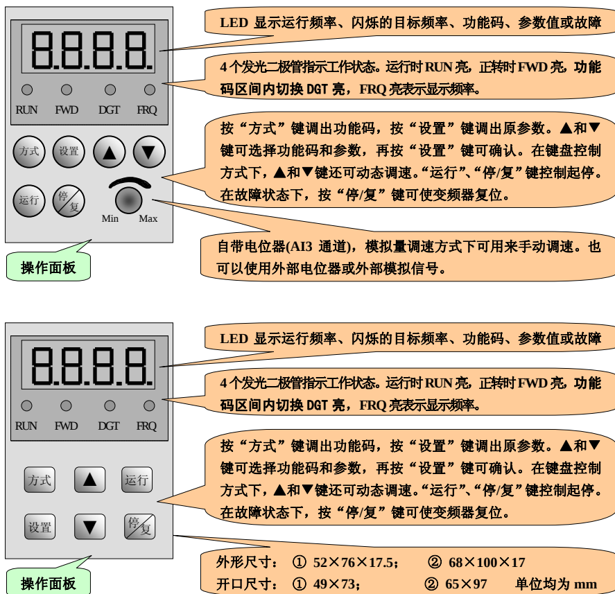
图 2-1 两种形式的操作面板
