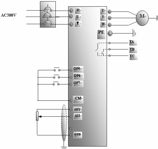
图 4-3 接线示意图 3
