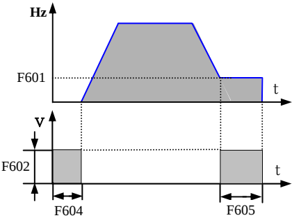
图 5-9 直流制动
