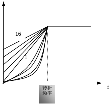
图 5-3 转矩提升示意图
