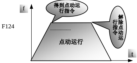
图 5-1 点动运行
