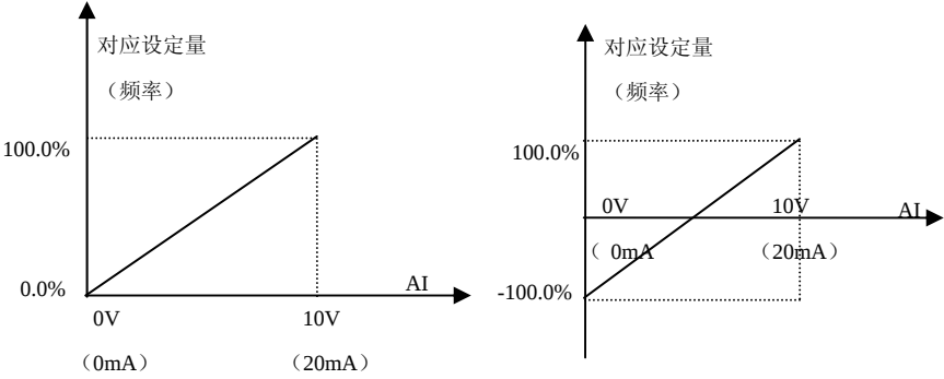
图 5-6 模拟给定与设定量的对应关系
