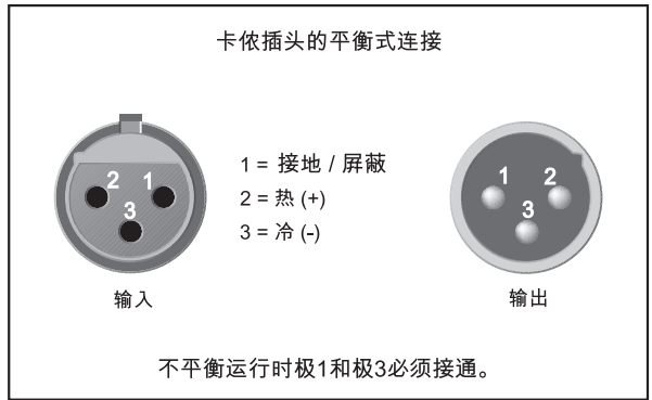
图 4. 3: 卡依插头
