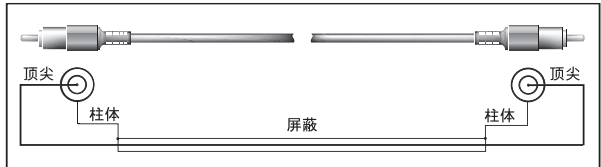
图 4. 4: “莲花” 电线
