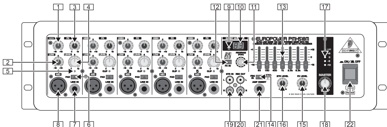
图 2.1: 面板上的控制元件和插口
