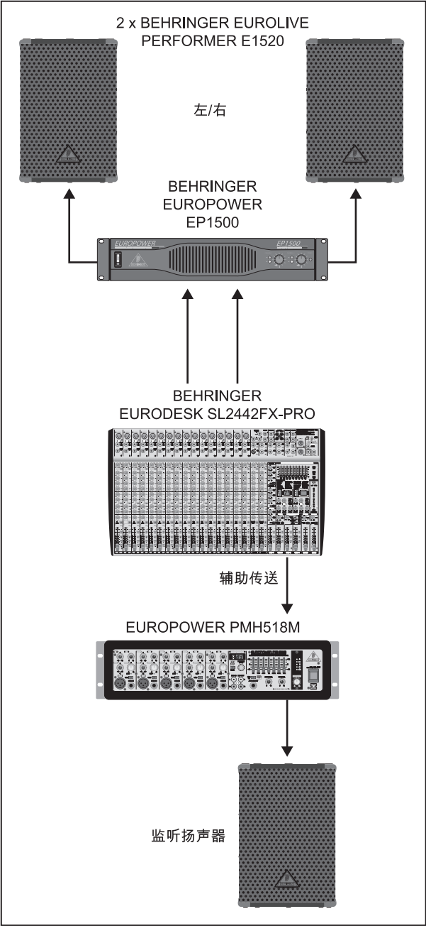
图 5.2: PMH518M 作为监听调音台使用时的连接
