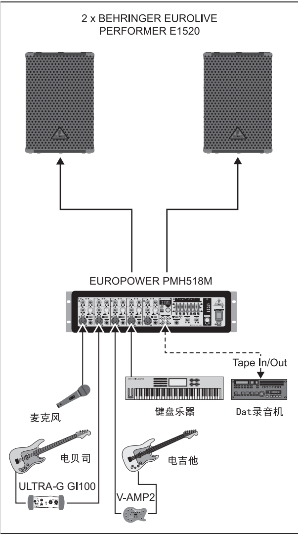
图 5. 1: 标准连接
