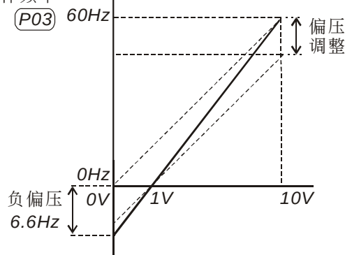
旋转VR时的对照图
