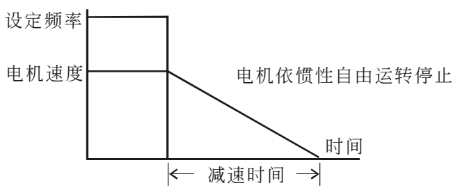
运转指令 ON OFF 图二：自由运转
