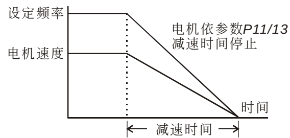
运转指令 ON OFF 图一：减速煞车
