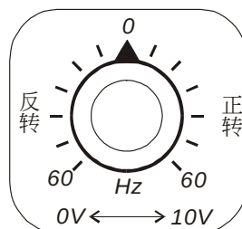
旋转VR时的对照图
