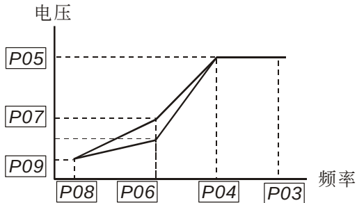
图三：特殊V/F曲线设定
