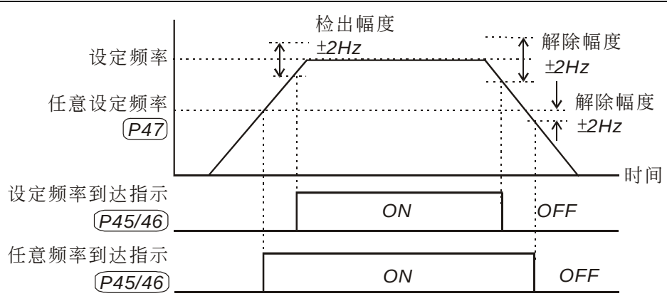
多机能端子频率到达输出对照图
