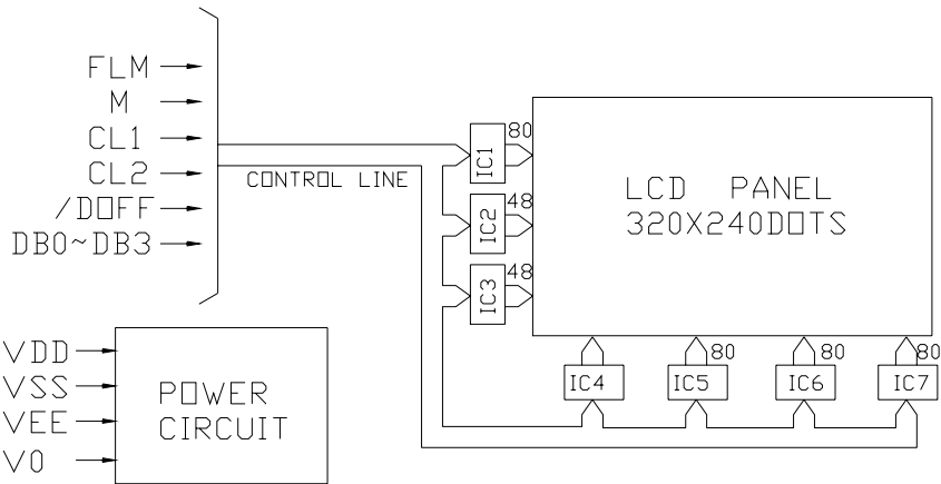
5-3. 电路图解
