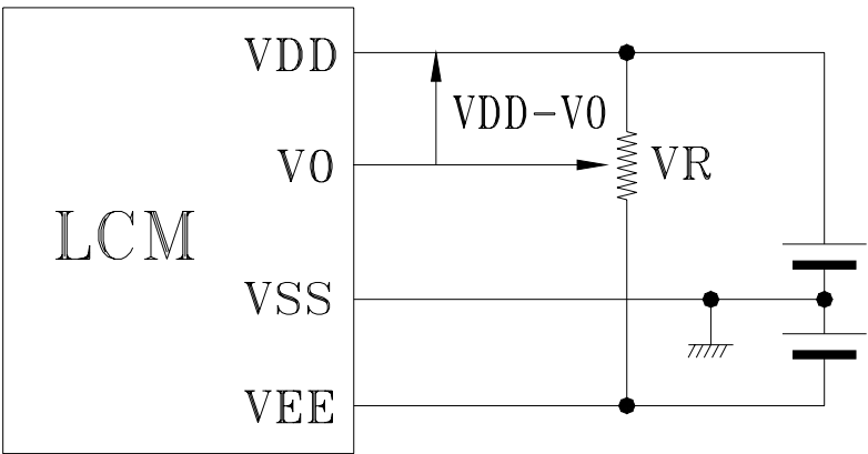
5-2. 电源连接图
