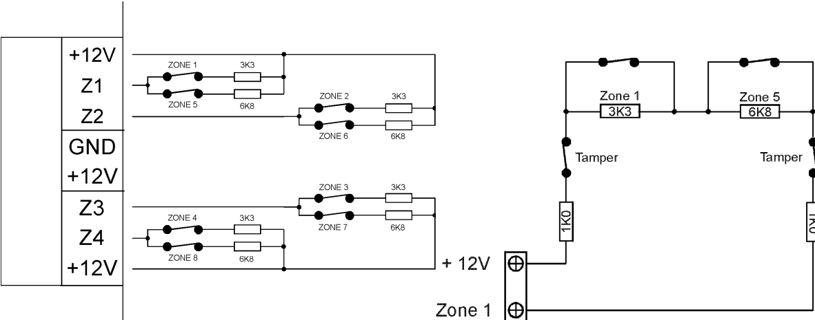
Figure 2: EOL 电阻接线图 (地址 266 = 15)
