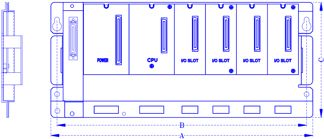
图 2-1 CPU 底板
